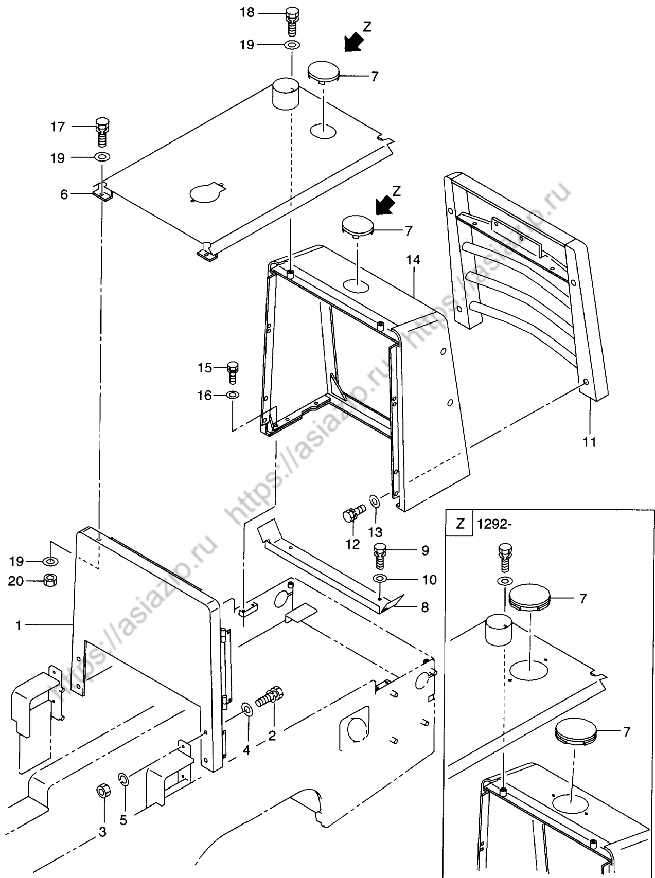
FIG. 105 HOOD & GRILLE (-2100) フード & グリル
