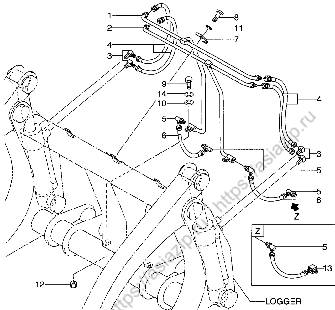
FIG. 160 LOGGER (PIPING) (TL047-648) ログ-（パイピング）
