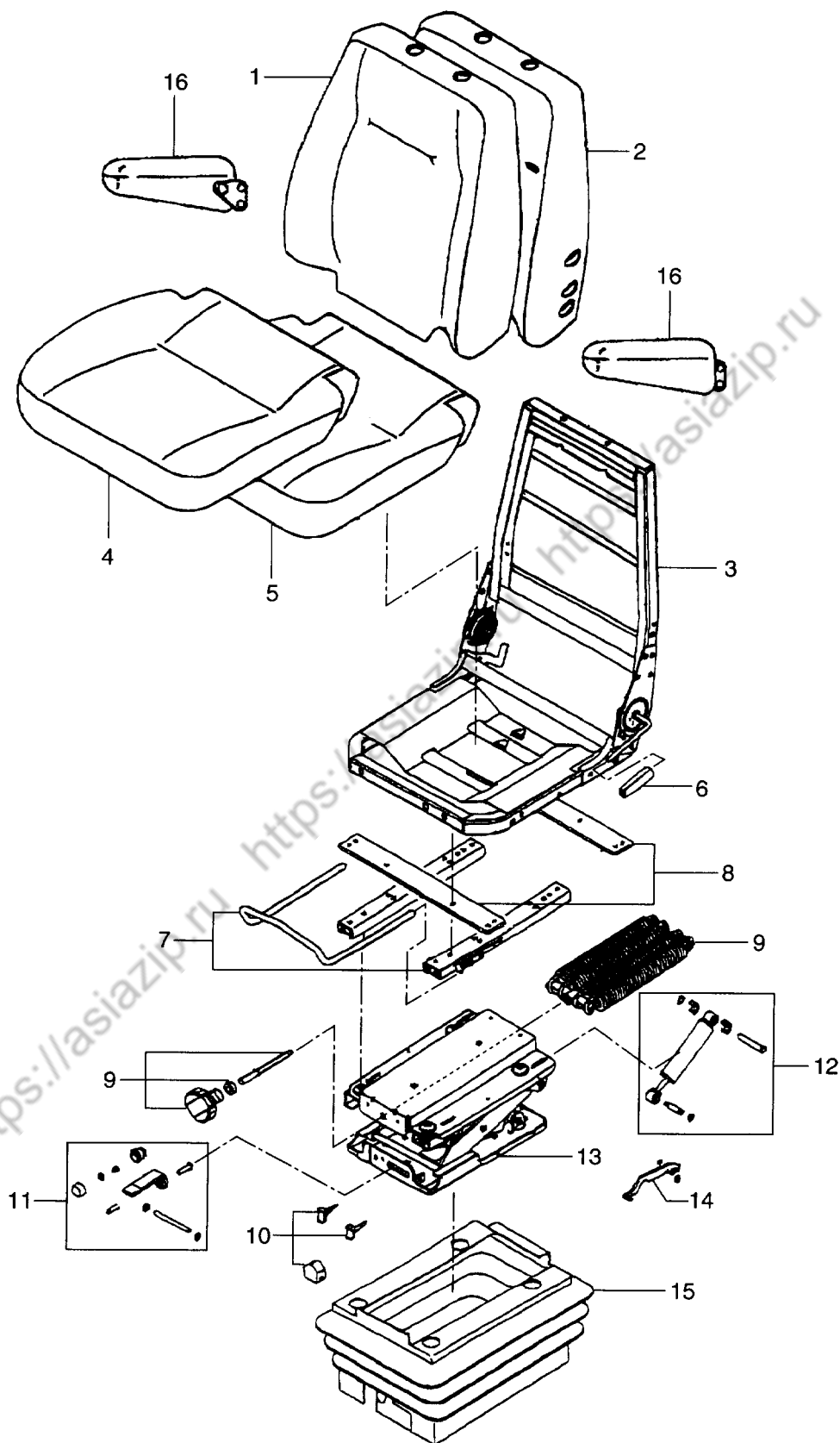
FIG. 73 SEAT (1356-) シート
