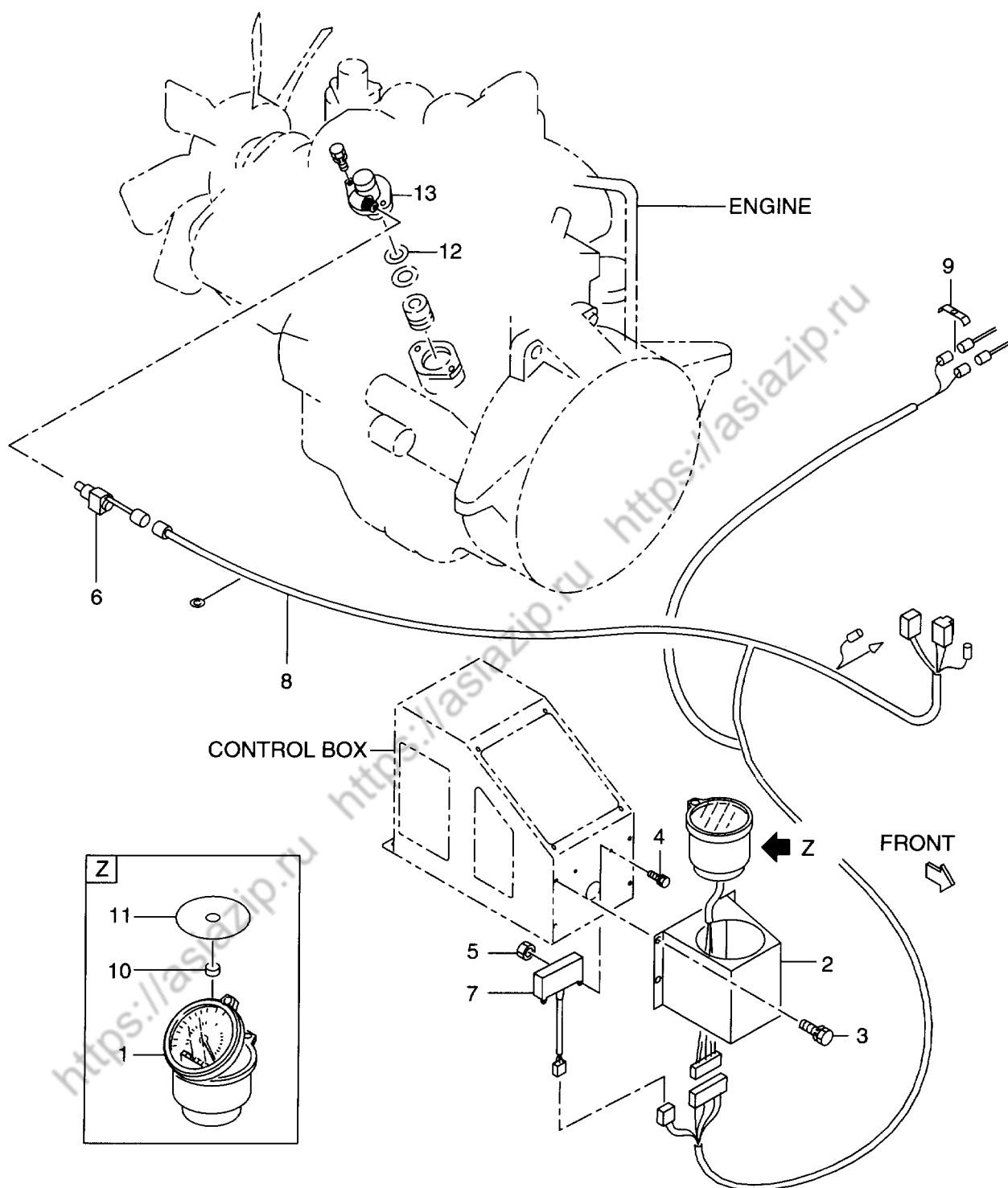
FIG. 32 TACHOGRAPH (TCO004-648) (OP) タコグラフ
