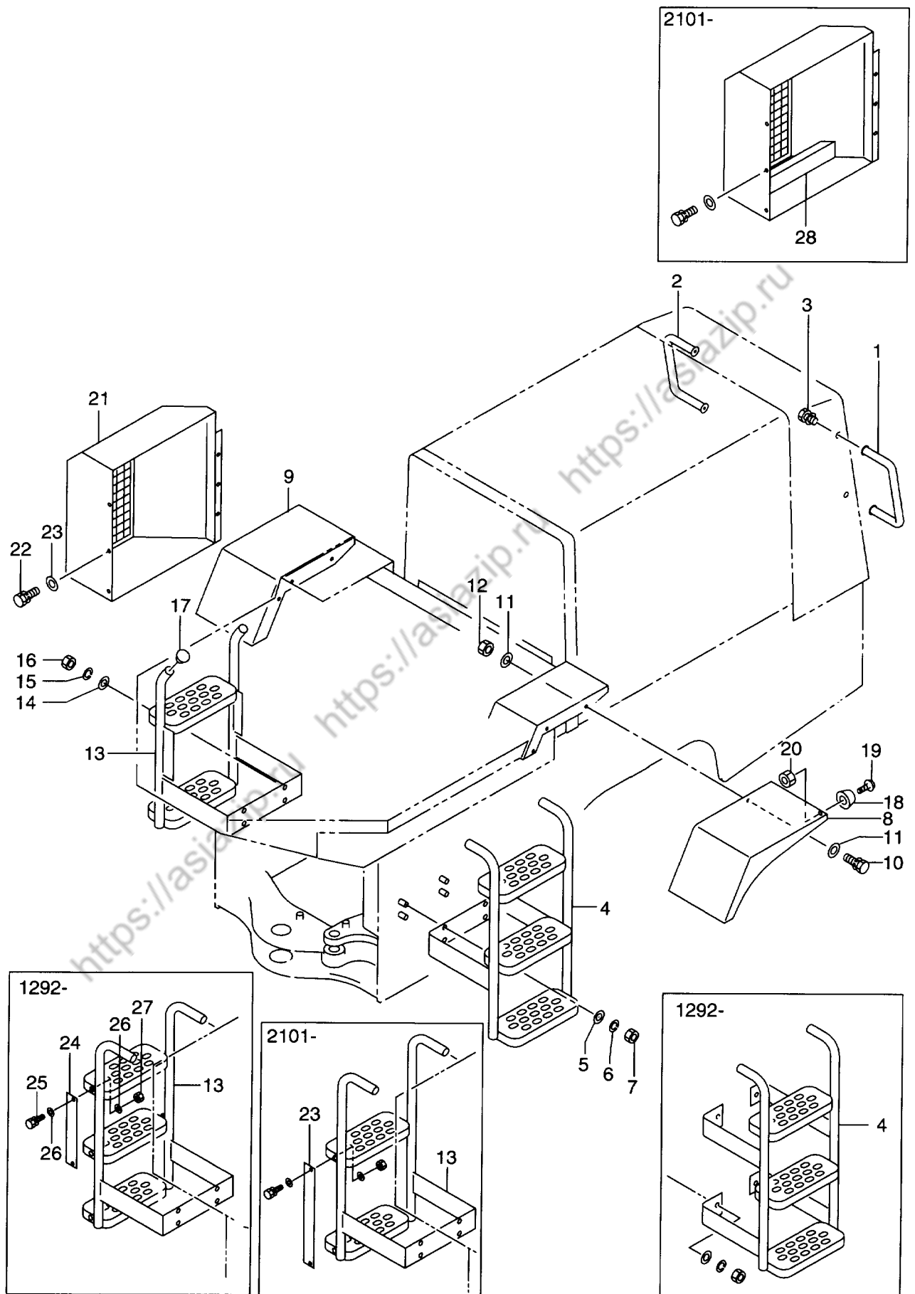
FIG. 108 STEP & REAR FENDER ステップ & リヤフェンダー
