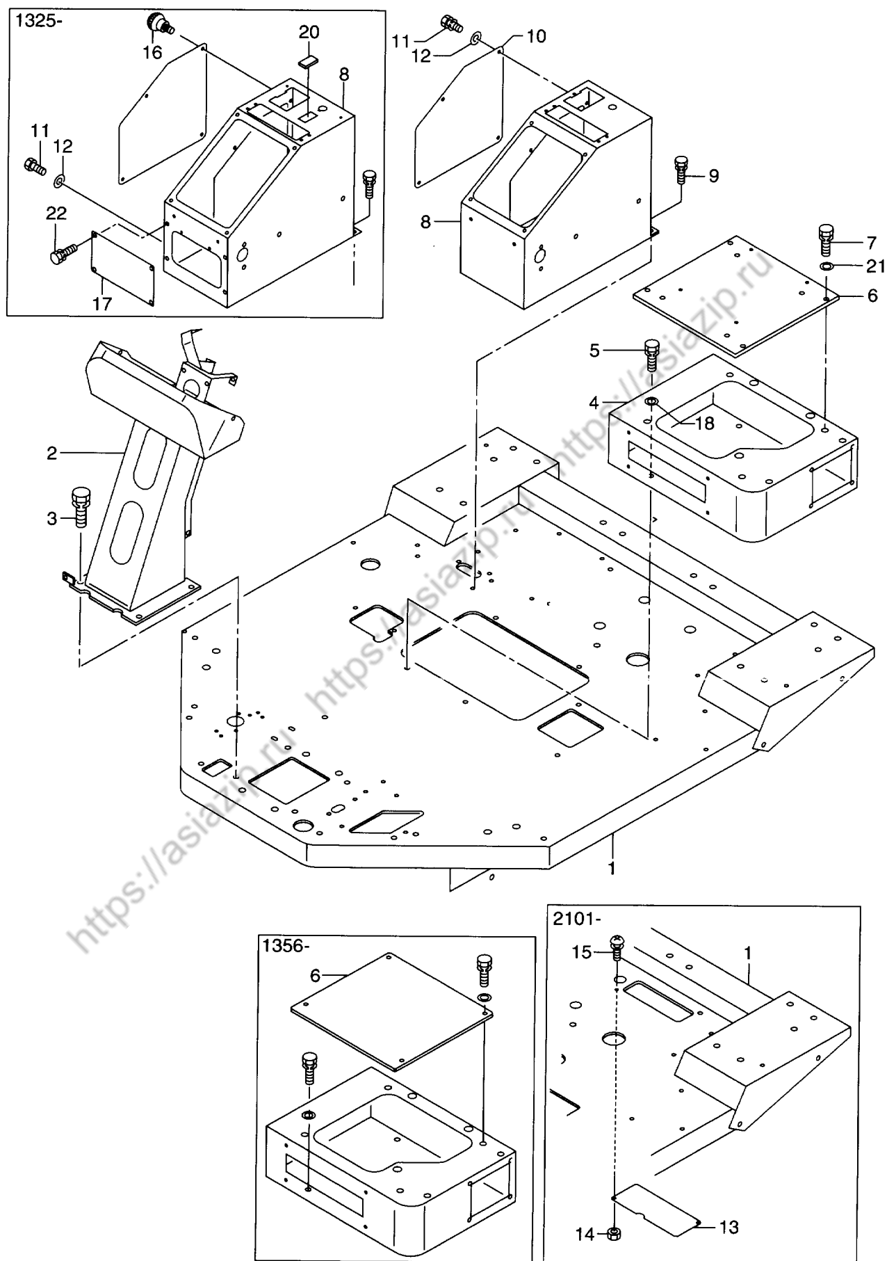
FIG. 71 COCKPIT コックピット
