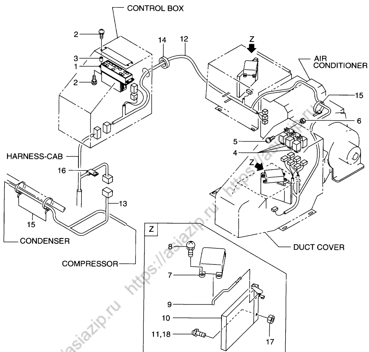
FIG. 154 AIR CONDITIONER (ELECTRICAL PARTS) イア-コンデ ィショナ(エレクトリカルパ ーツ)
