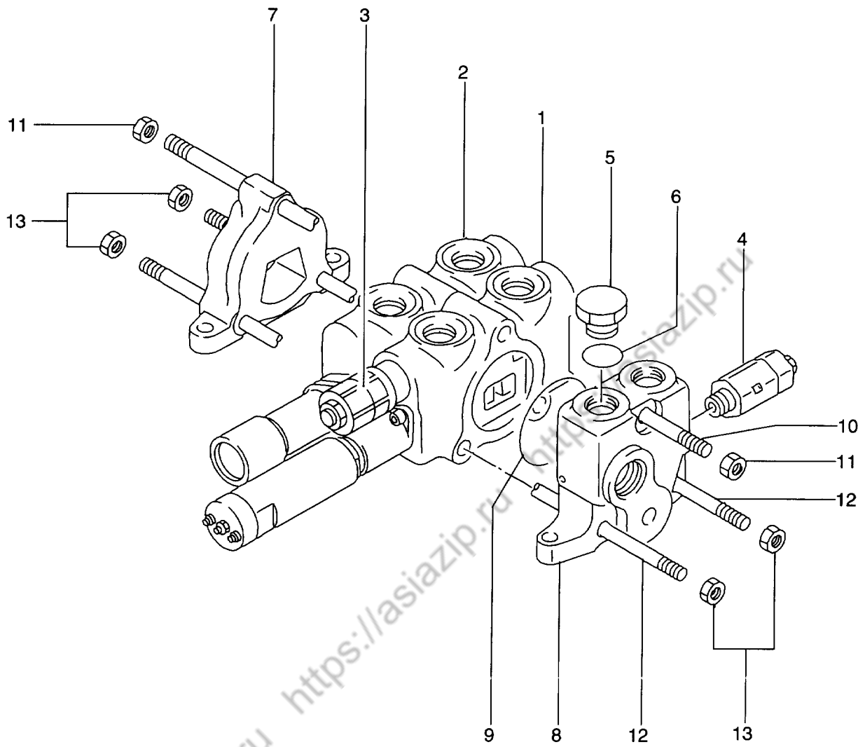
FIG. 118 CONTROL VALVE コントロールバルブ
