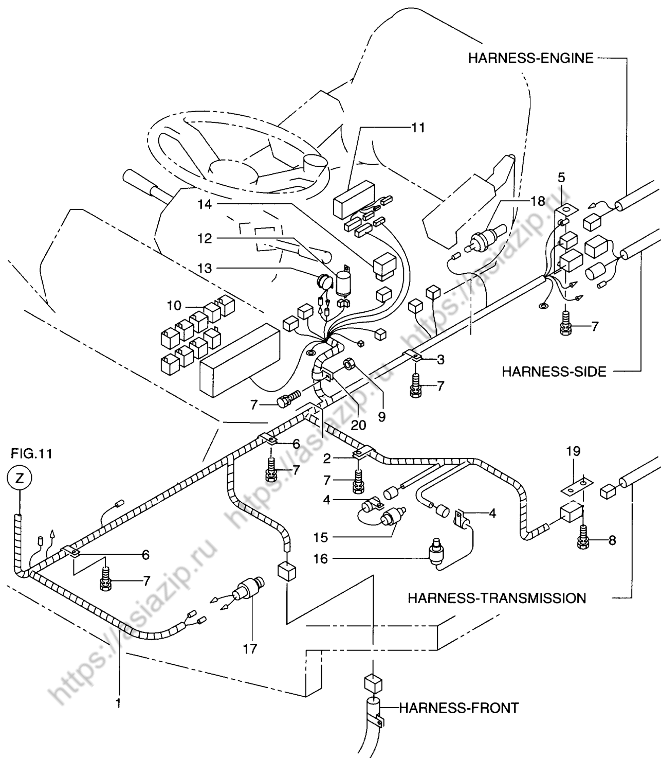
FIG. 10A WIRING (COCKPIT) (1/2) (2101-) ワイヤリング (コックピット)
