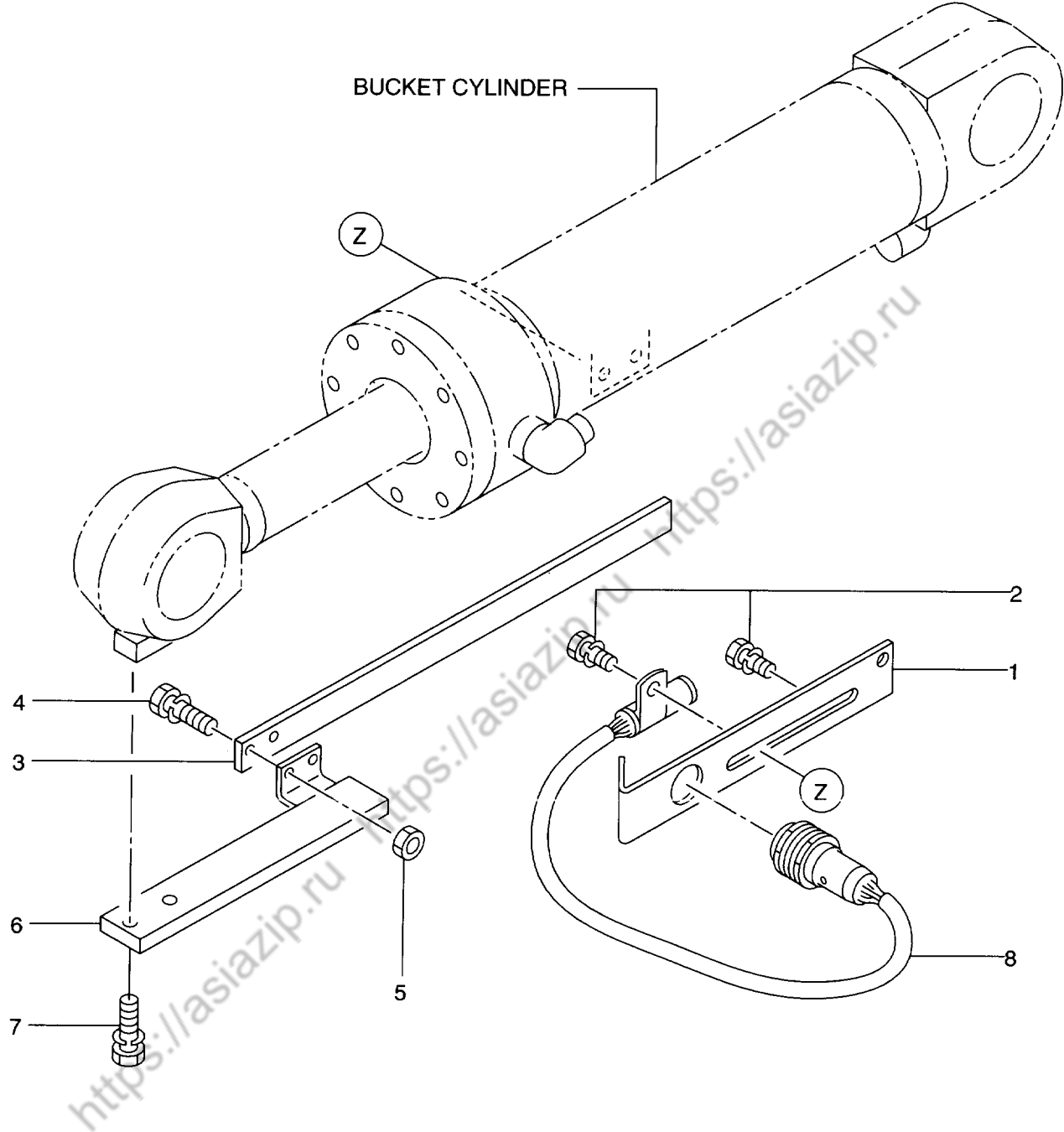
FIG. 149 BUCKET LEVELER バケットレベラ
