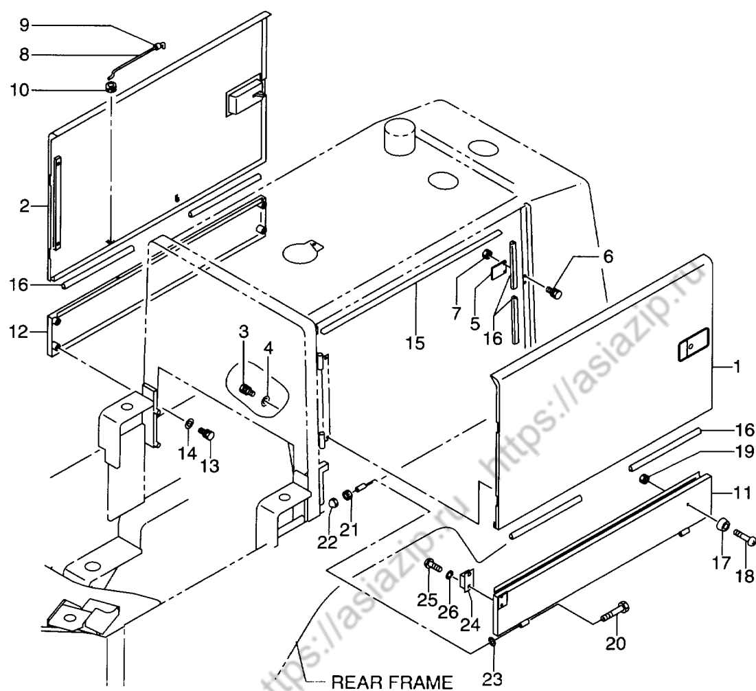
FIG. 106 SIDE PANEL サイドパネル
