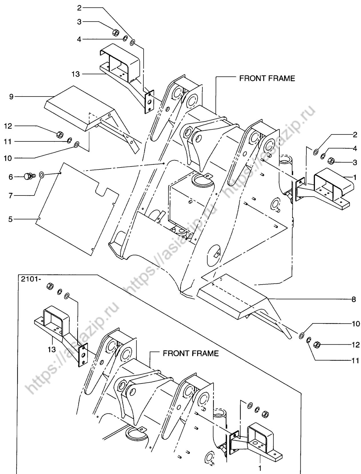
FIG. 107 LAMP BRACKET & FRONT FENDER ランプブラケット&フロントフェンダー
