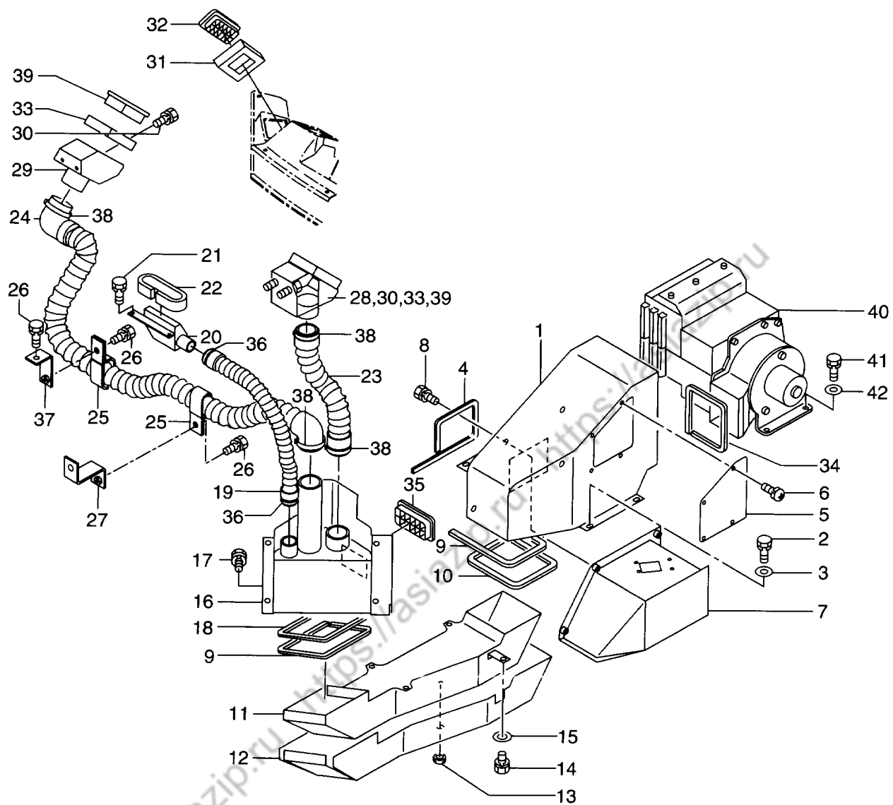
FIG. 150A AIR CONDITIONER (1/2) (2101-) エア-コンディショナ
