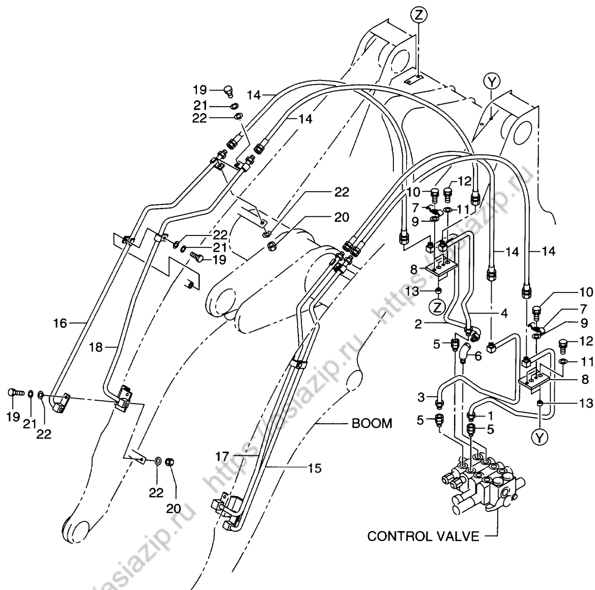
FIG. 124 PIPING KIT WITH 4 SPOOL VALVE (PIPING) (AP4002-648) (OP) 4連バルブ付パ〇化〇ンクキット(パ〇化〇ンク)
