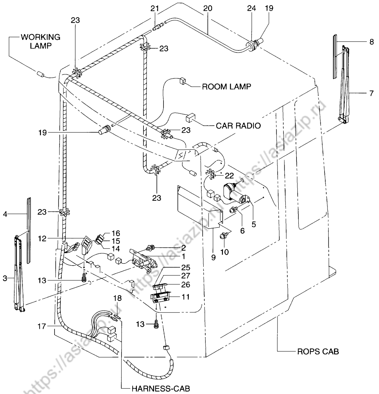
ROPS CAB (WIPER) 〇フ° スキャブ° (ワイバ°)
