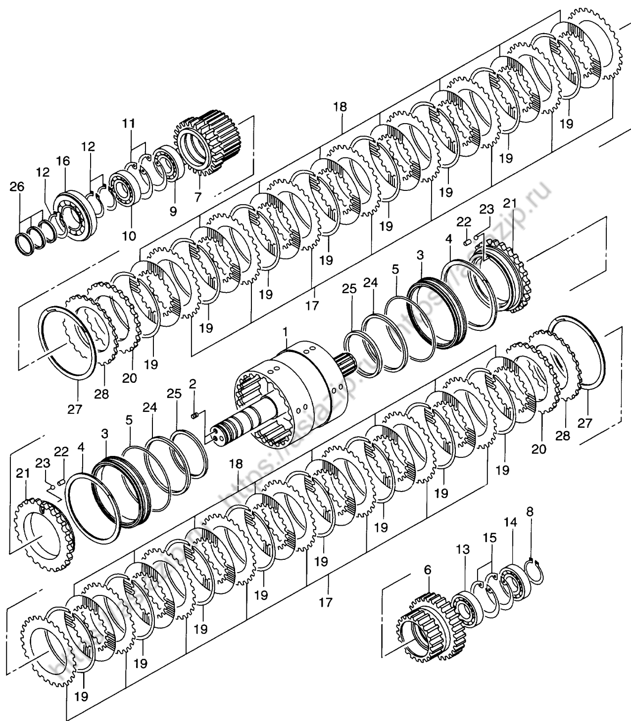
FIG. 39 CLUTCH (FORWARD & REVERSE) クラッチ(フォワード & リバース)
