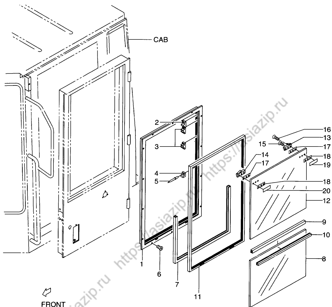
FIG. 99 CAB (DOOR, LH) (1/2) (LCB150-648) (OP) キャブ (ドア)
