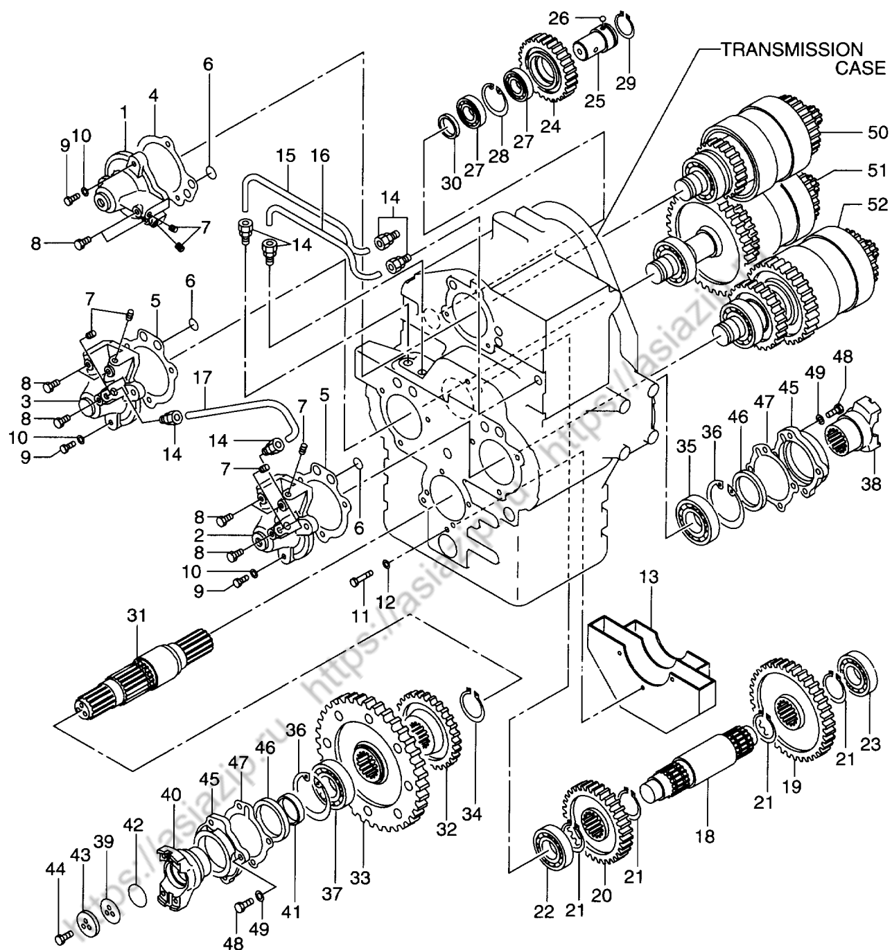
FIG. 35 DRIVE UNIT (2/3) ドライブユニット
