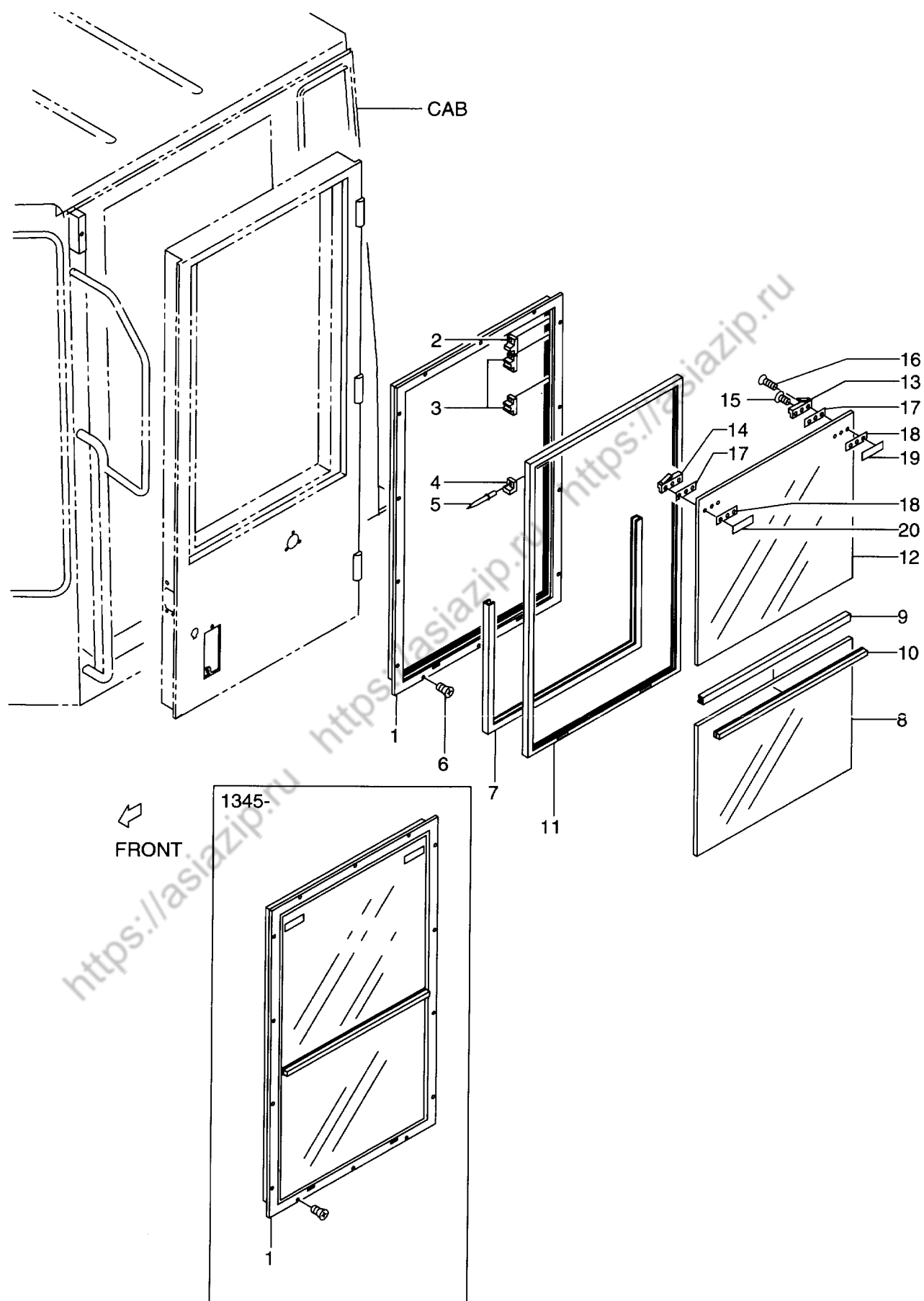
FIG. 89 CAB (DOOR, LH) (1/2) (SCB001-648) (OP) キャブ (ドア-)
