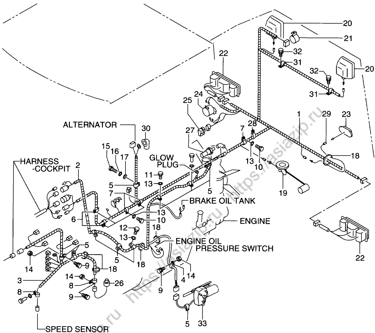
FIG. 12 WIRING (REAR FRAME) (-2100) ワイヤリング (リヤ-フレーム)
