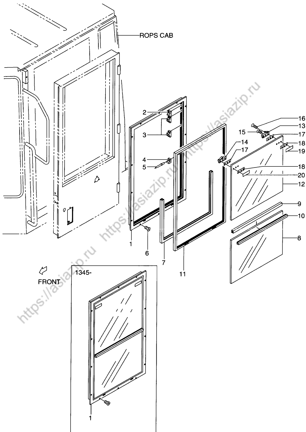
FIG. 79 ROPS CAB (DOOR,LH) (1/2) ロフ° スキャブ (ドア-)
