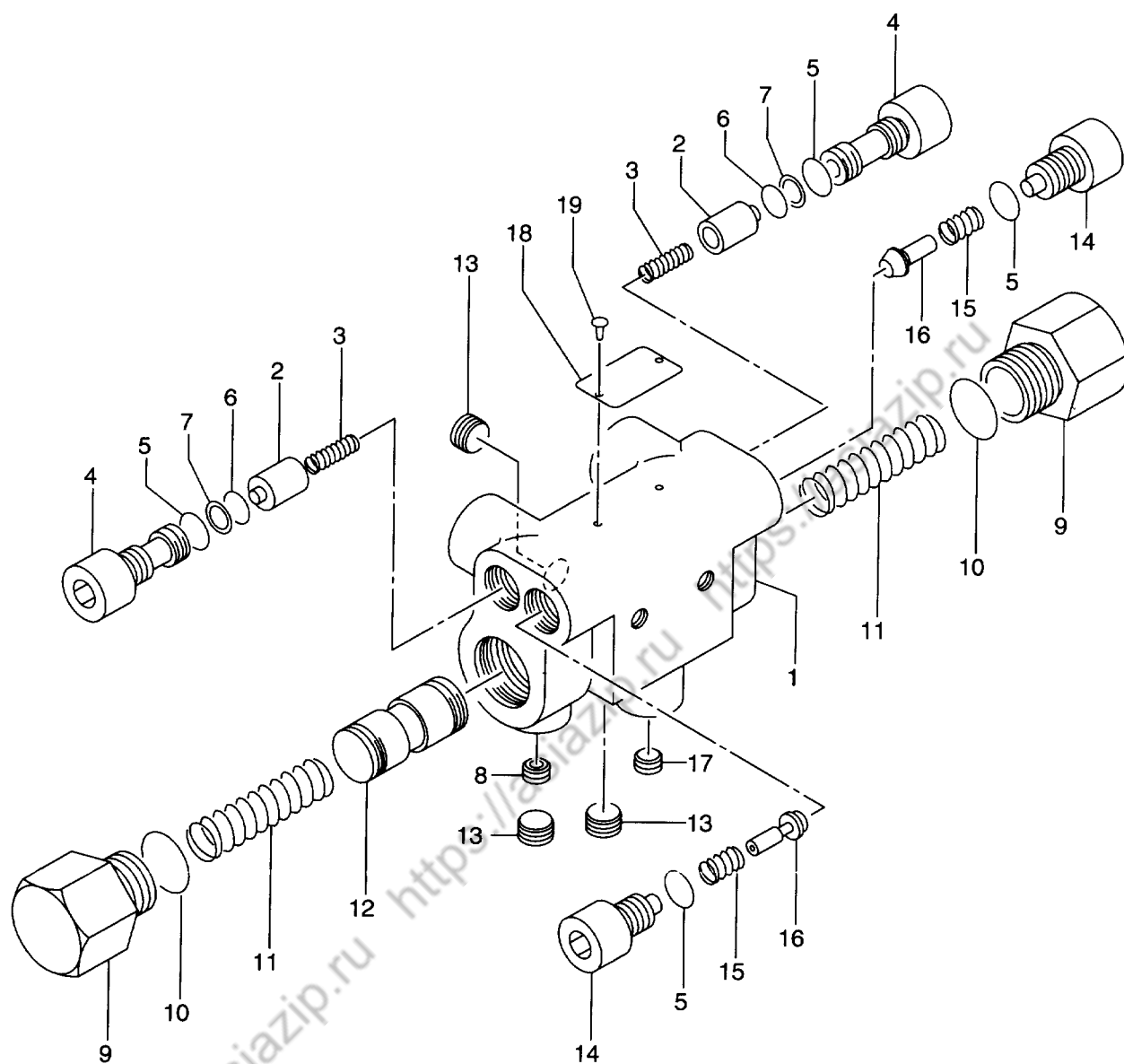
FIG. 135 CUSHION VALVE クッションバルブ
