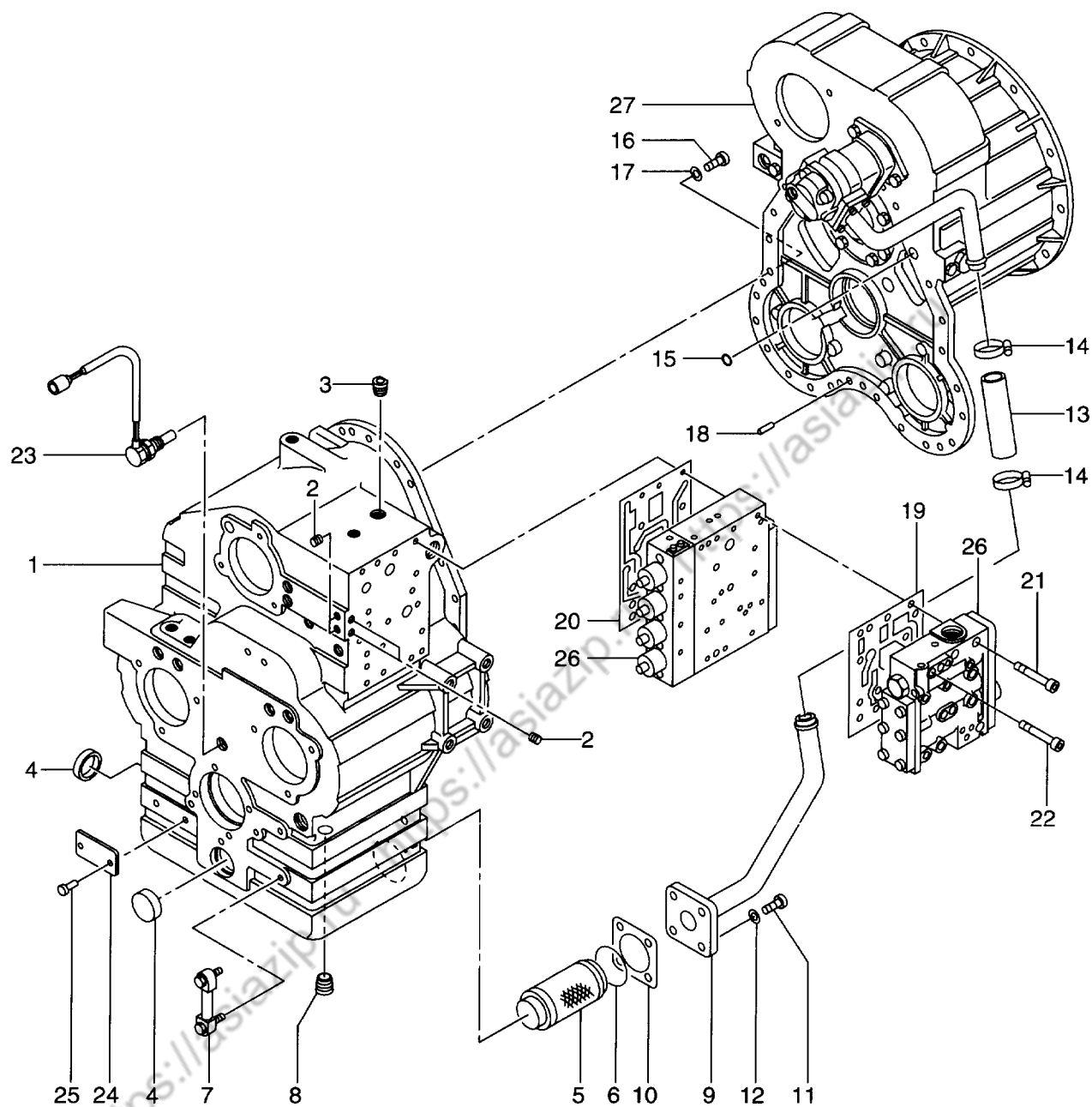
FIG. 34 DRIVE UNIT (1/3) ドライブユニット
