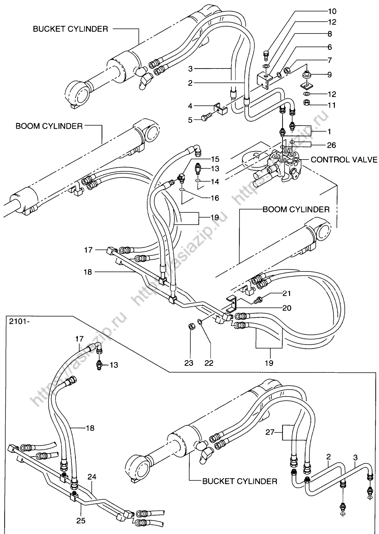
FIG. 133 HYDRAULIC LINE (BOOM & BUCKET) ハイドロリックライン(ブーム&バケット)
