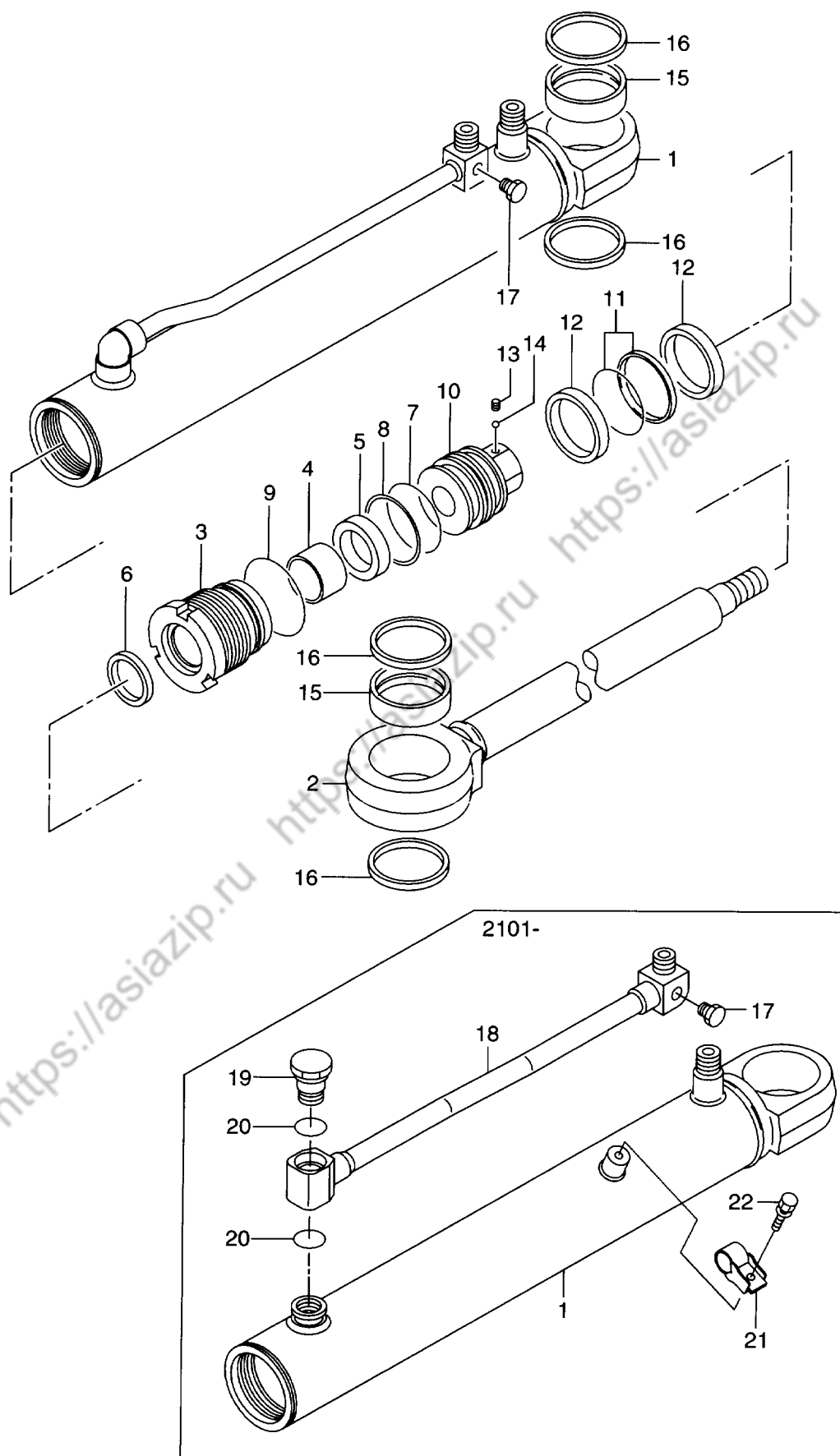
FIG. 67 STEERING CYLINDER ステアリング シリンダ
