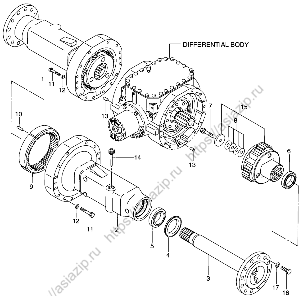
FIG. 49 DRIVE AXLE - REAR (1/3) ドライブアクスル(リヤー)
