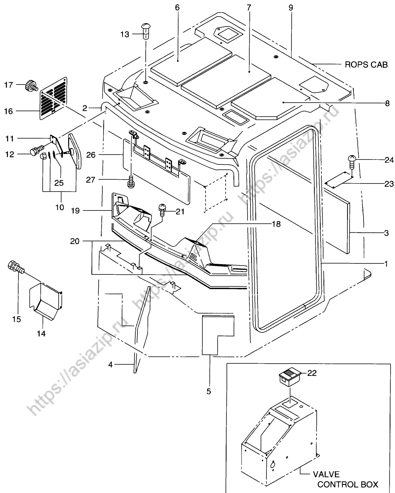
FIG. 76 ROPS CAB (COVER & MAT) ロブスカブ (カバー&マット)
