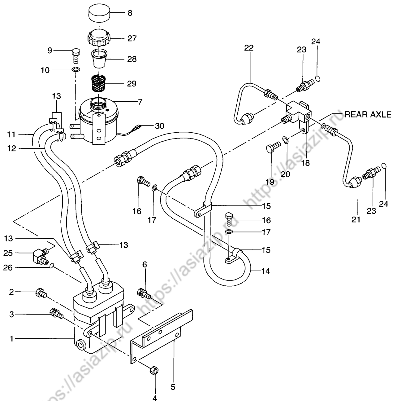
FIG. 60 BRAKE LINE (SPLIT CYLINDER - REAR AXLE) ブレーキライン(スプリットシリンダー-リヤ-アクスル)
