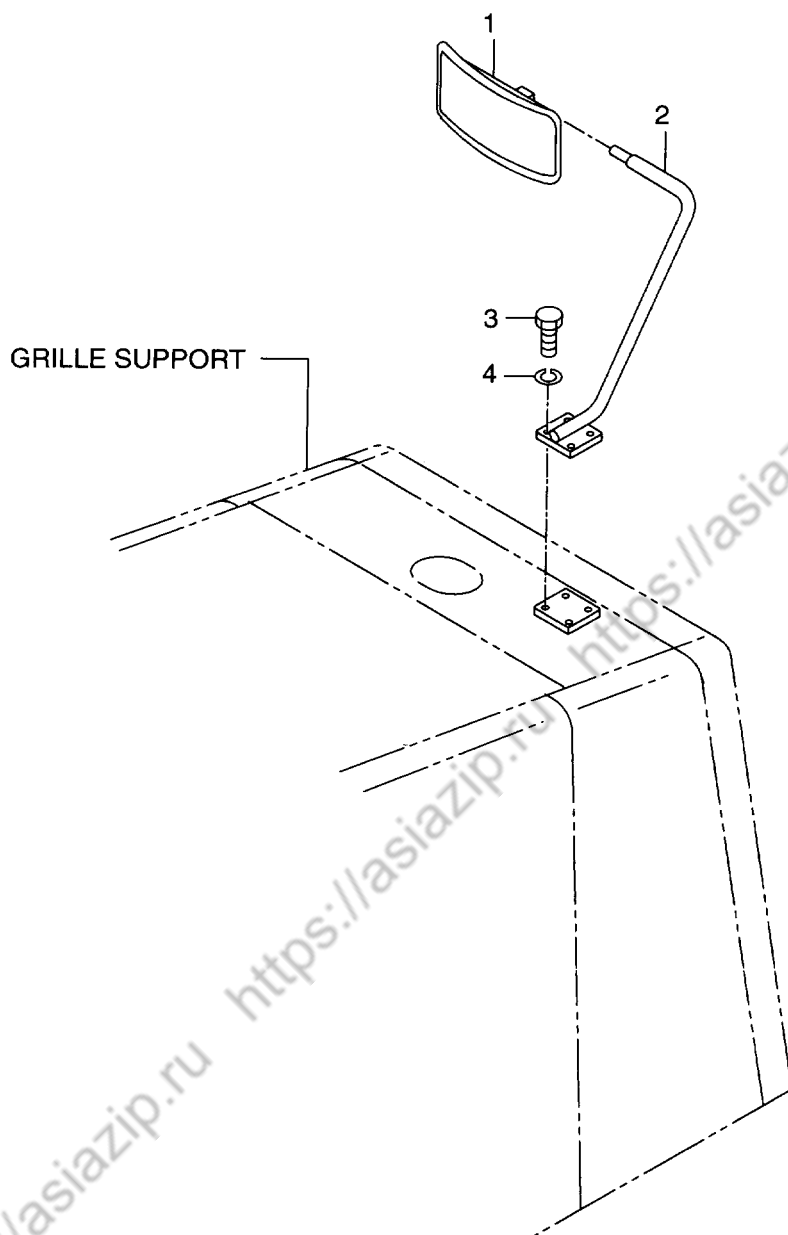
FIG. 115 UNDER MIRROR (UMR001-648) (OP) アンダーミラー
