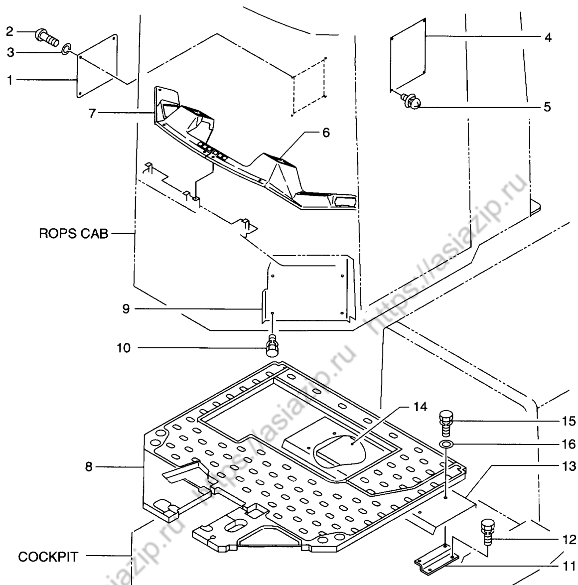
FIG. 111 AIR-CON LESS KIT(DASHBOARD & MAT)(ACLS3-648)(OP) エア-コンデ ィションナレスキット(ダ ッッシュボード & マット)
