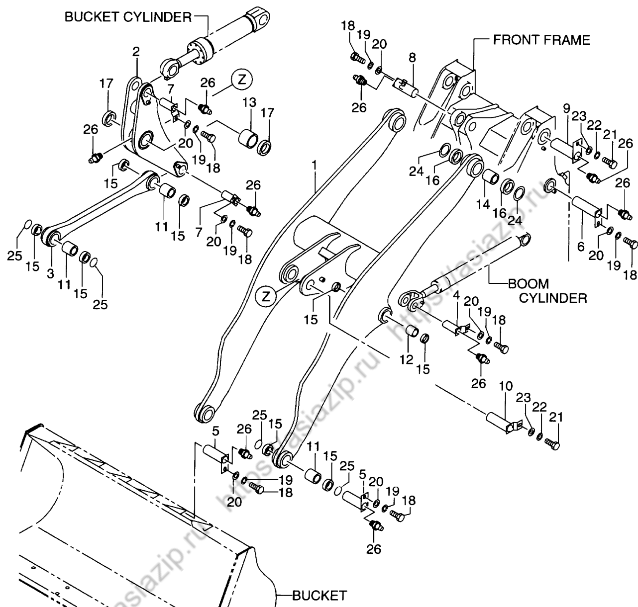
FIG. 137 BOOM 7-4
