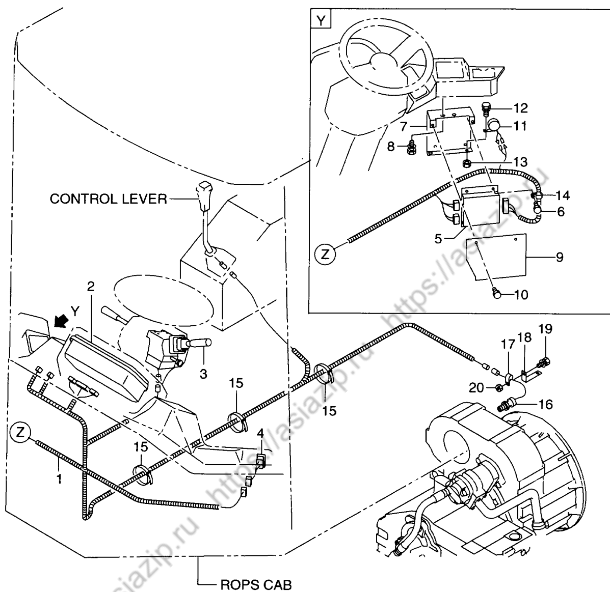
FIG. 26 AUTOMATIC TRANSMISSION (ATM-648) (OP) オートマチックトランスミッション
