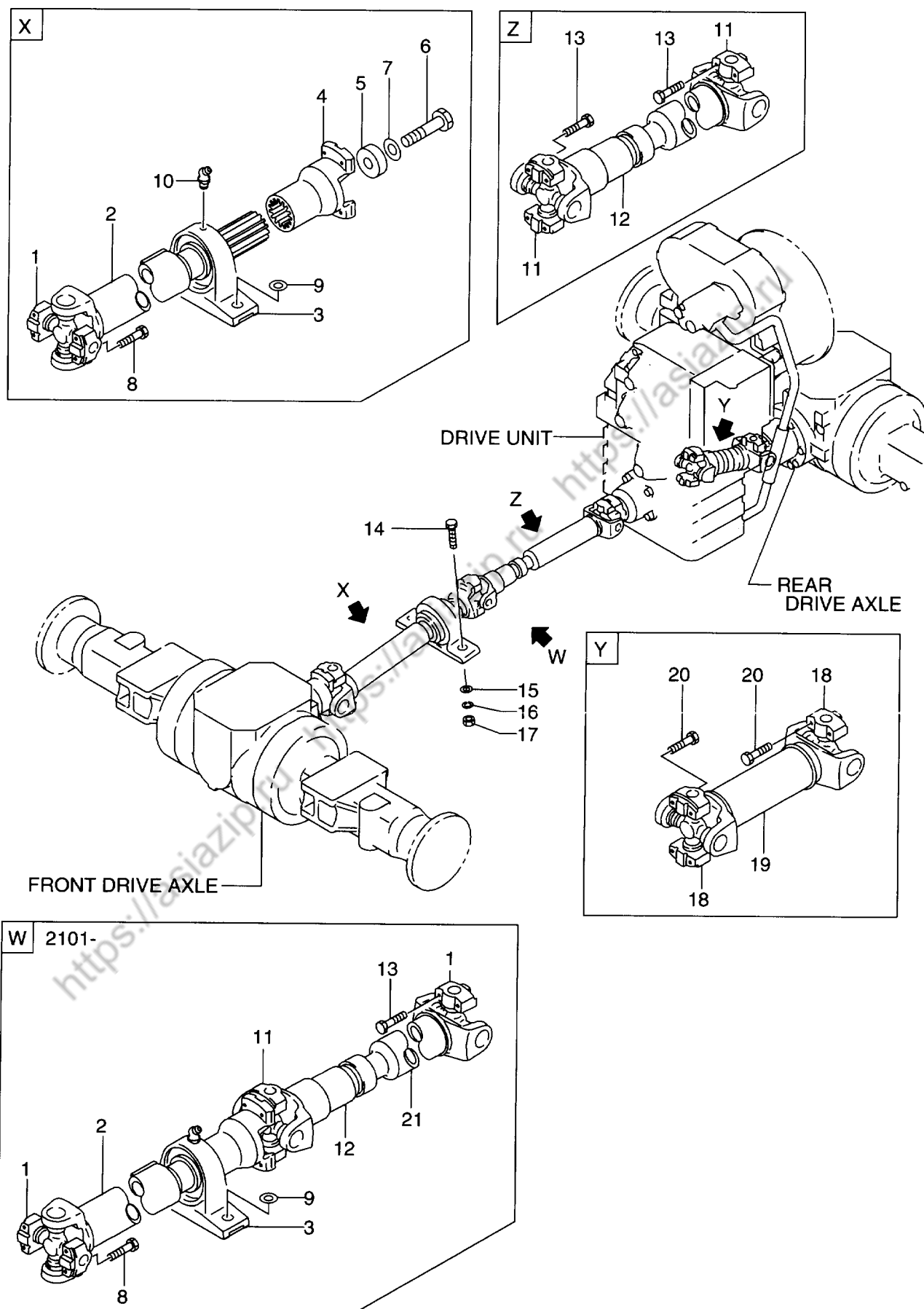
FIG. 55 PROPELLER SHAFT プロペラシャフト
