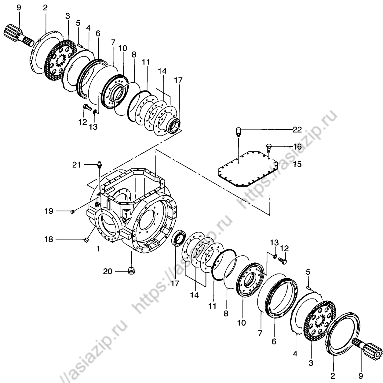
FIG. 50 DRIVE AXLE - REAR (2/3) ドライブアクスル(リヤー)
