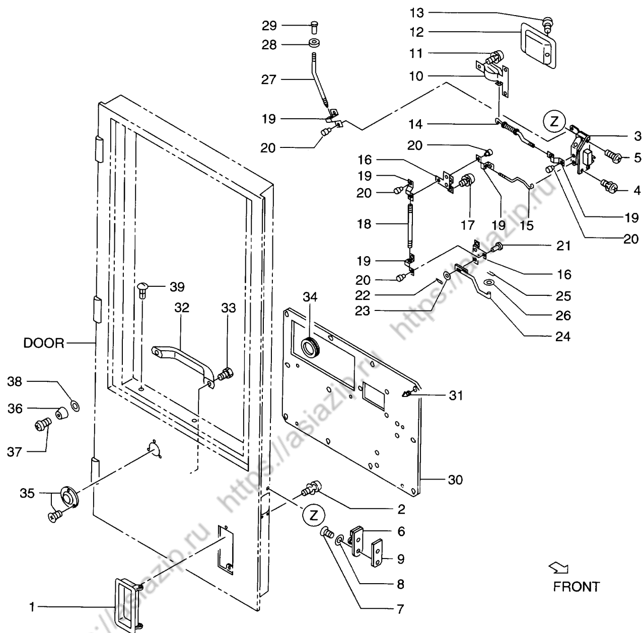
FIG. 88 CAB (DOOR, RH) (2/2) (SCB001-648) (OP) キャブ(ドア-)
