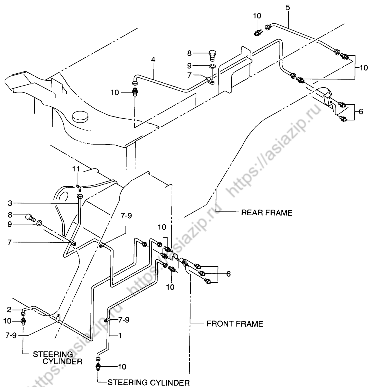
FIG. 155 GREASE PIPING グリースパイピング
