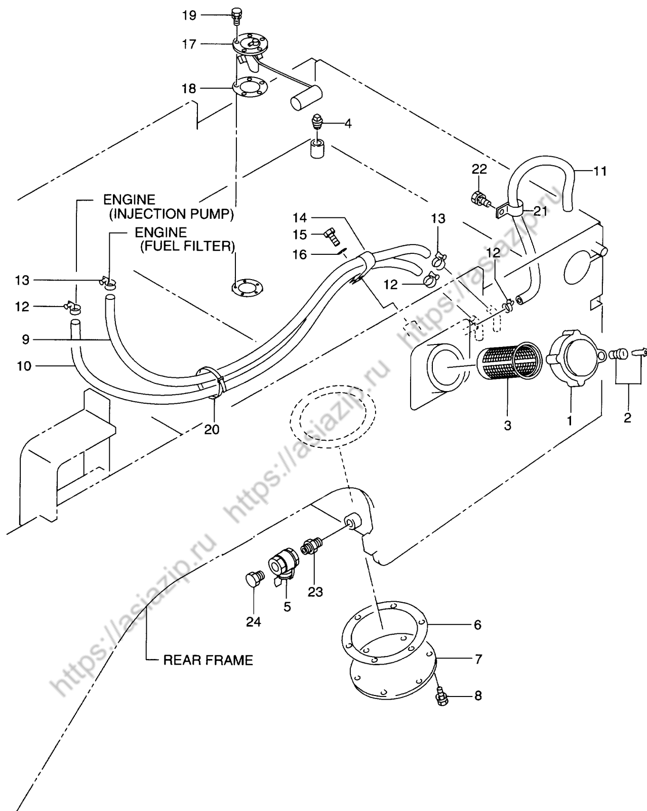
FIG. 6 FUEL SYSTEM (-2100) フューエルシステム
