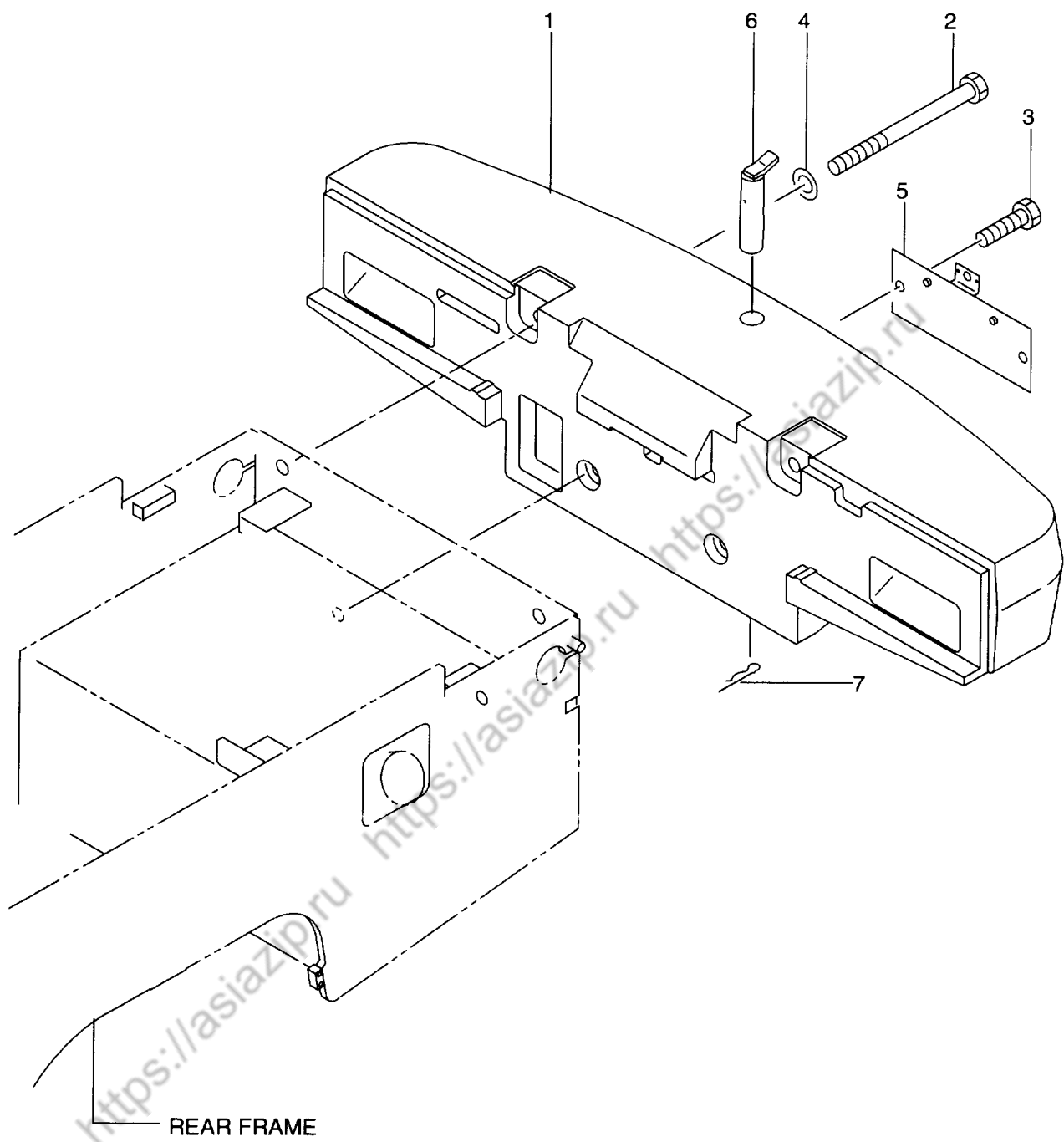
FIG. 70 BALANCE WEIGHT バ ラ ンス ウ ェ イ ト
