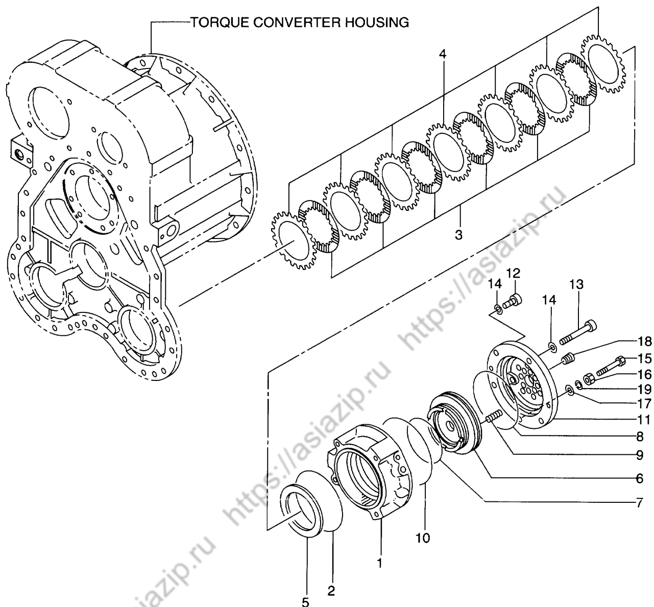
FIG. 36 DRIVE UNIT (3/3) ドライブユニット
