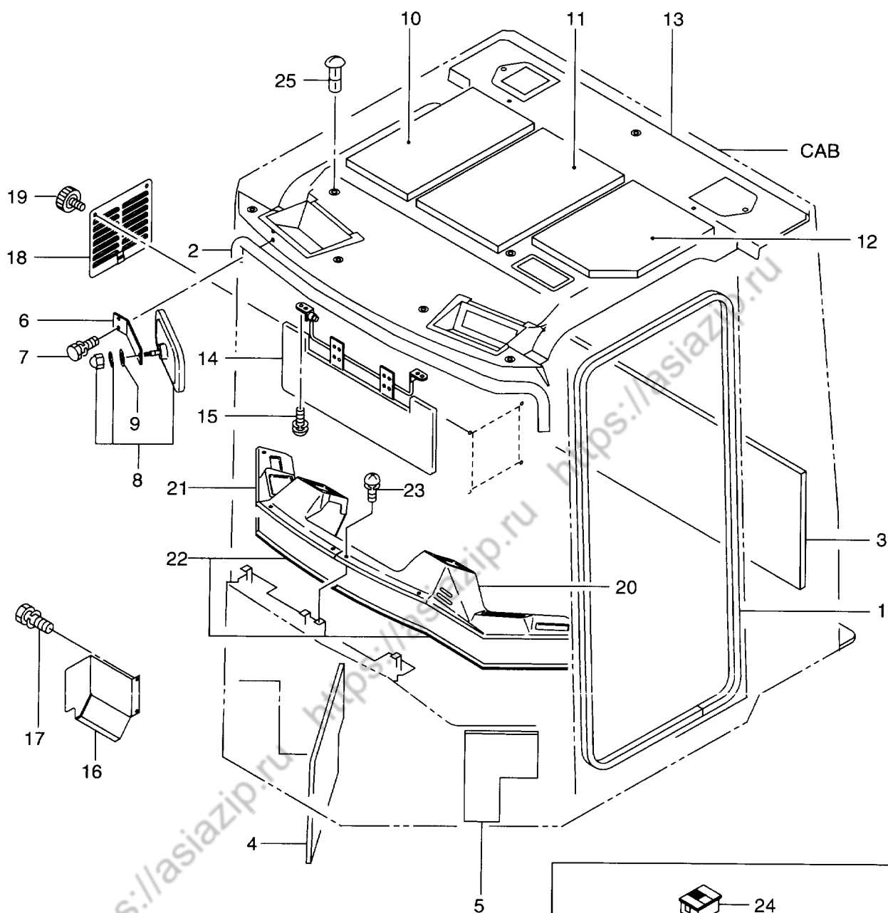
FIG. 86 CAB (COVER & MAT) (SCB001-648) (OP) キャブ (カバー&マット)
