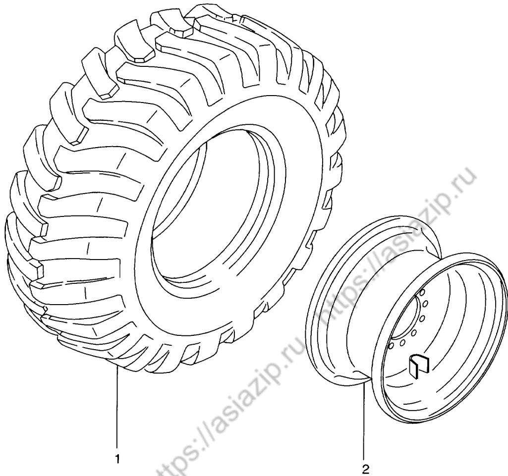
FIG. 53 WHEEL ホイール
