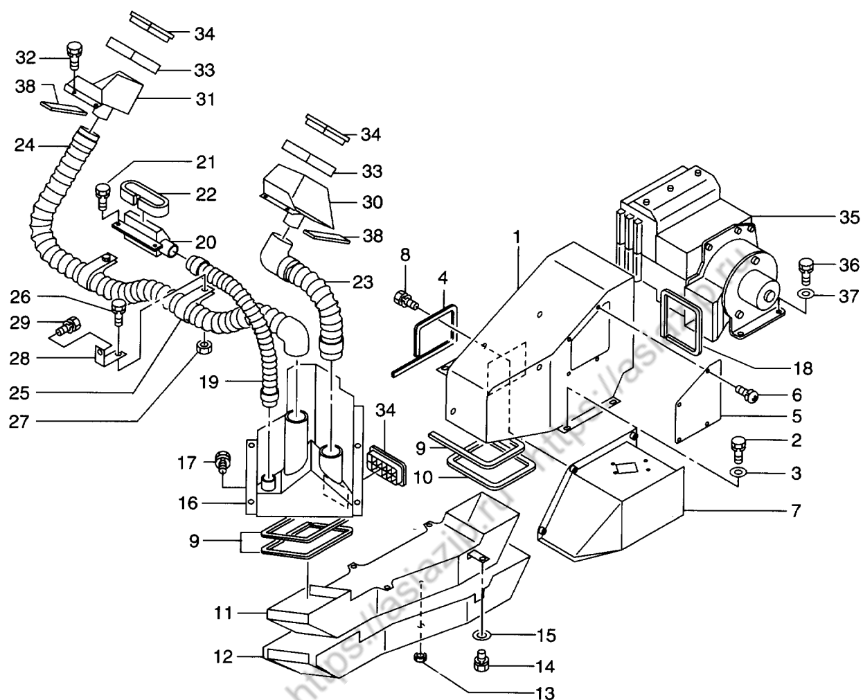
FIG. 150 AIR CONDITIONER (1/2) (-2100) イア-コンデ イショナ
