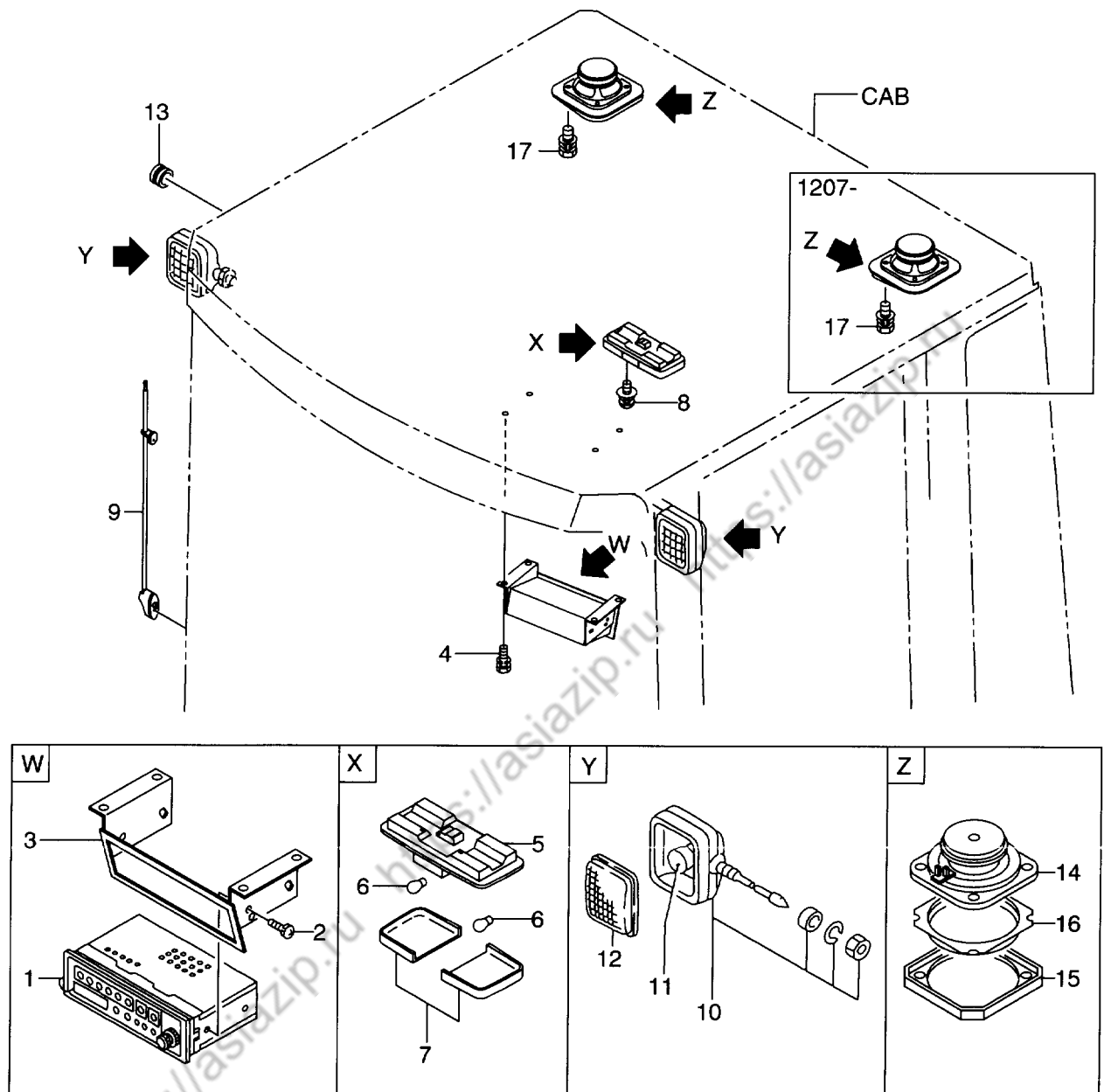
FIG. 101 CAB (LAMP & RADIO) (LCB150-648) (OP) キャブ (ランプ & ラジオ)
