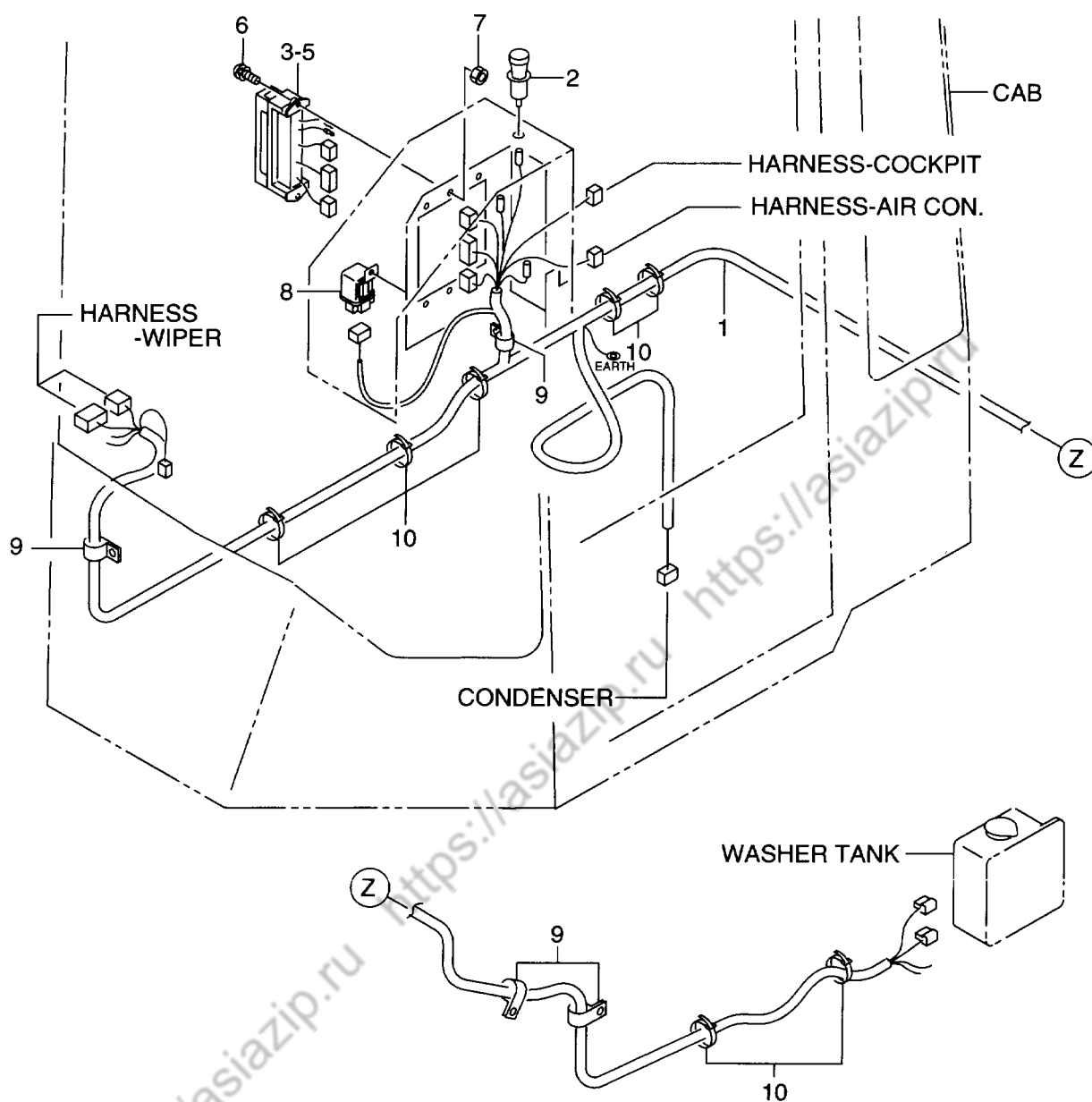
FIG. 93 CAB (ELECTRICAL) (SCB001-648) (OP) キャブ (エレクトリカル)
