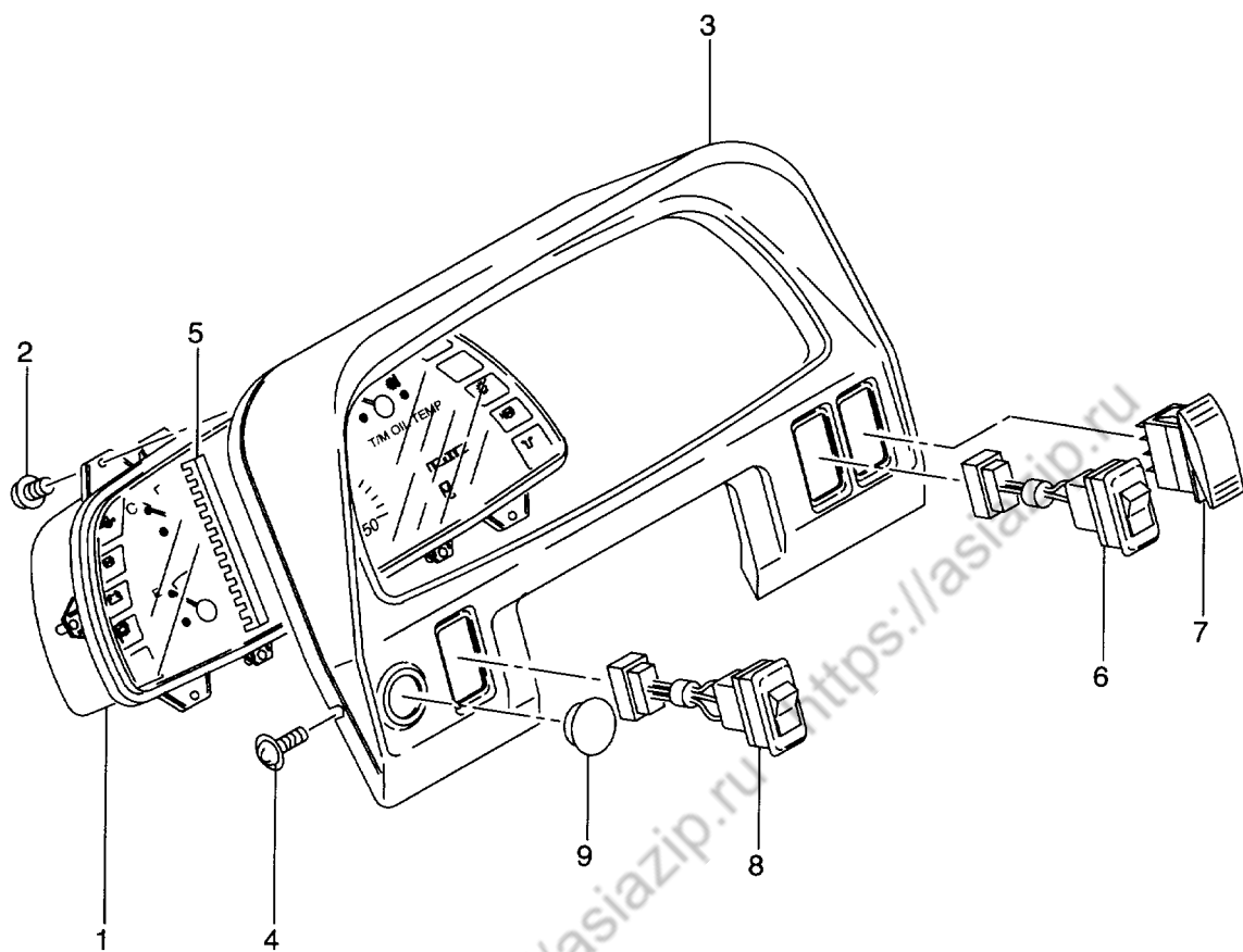
FIG. 15 INSTRUMENT PANEL インストルメントパネル
