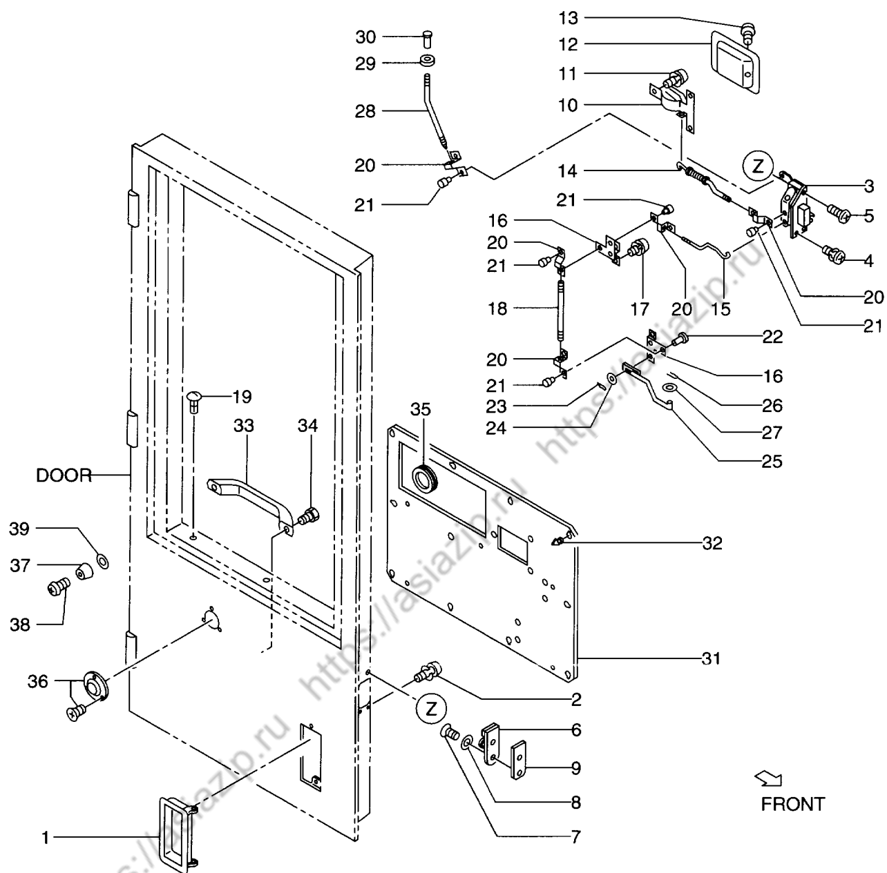
FIG. 78 ROPS CAB (DOOR,RH) (2/2) ロフスカブ(ドア-)
