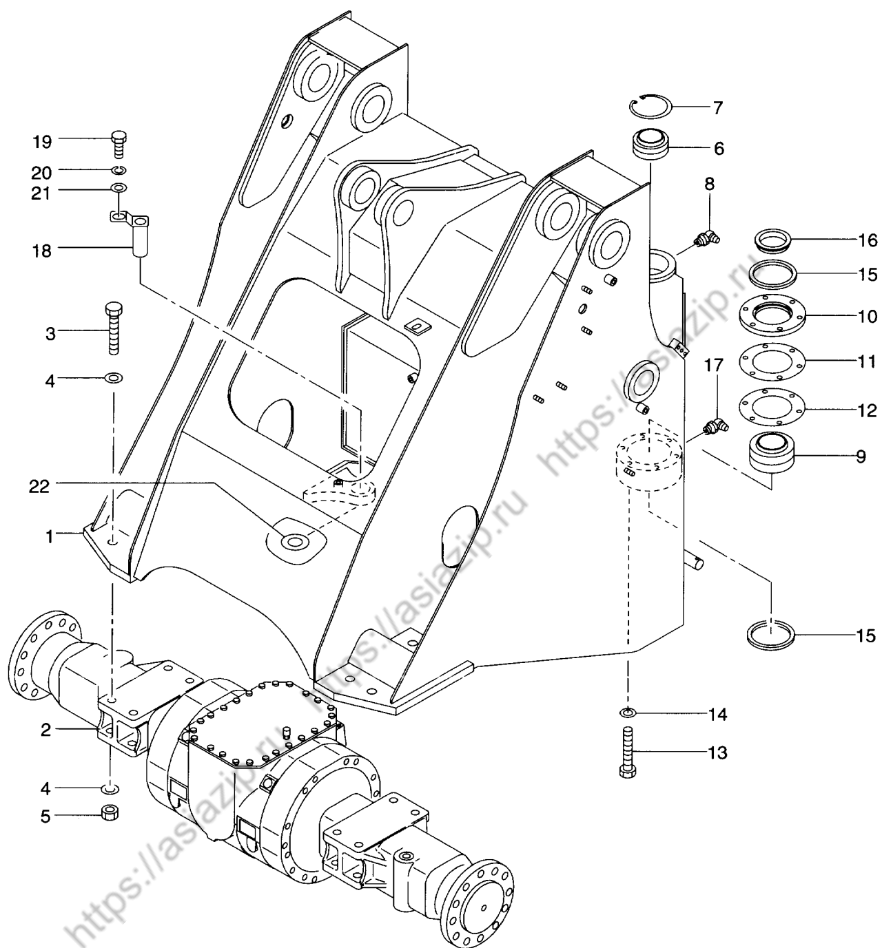
FIG. 68 FRONT FRAME フロントフレーム
