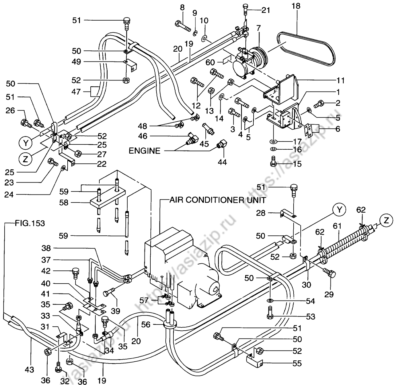
FIG. 152 AIR CONDITIONER PIPING (1/2) イア-コンデ イショナ°化°ン°グ
