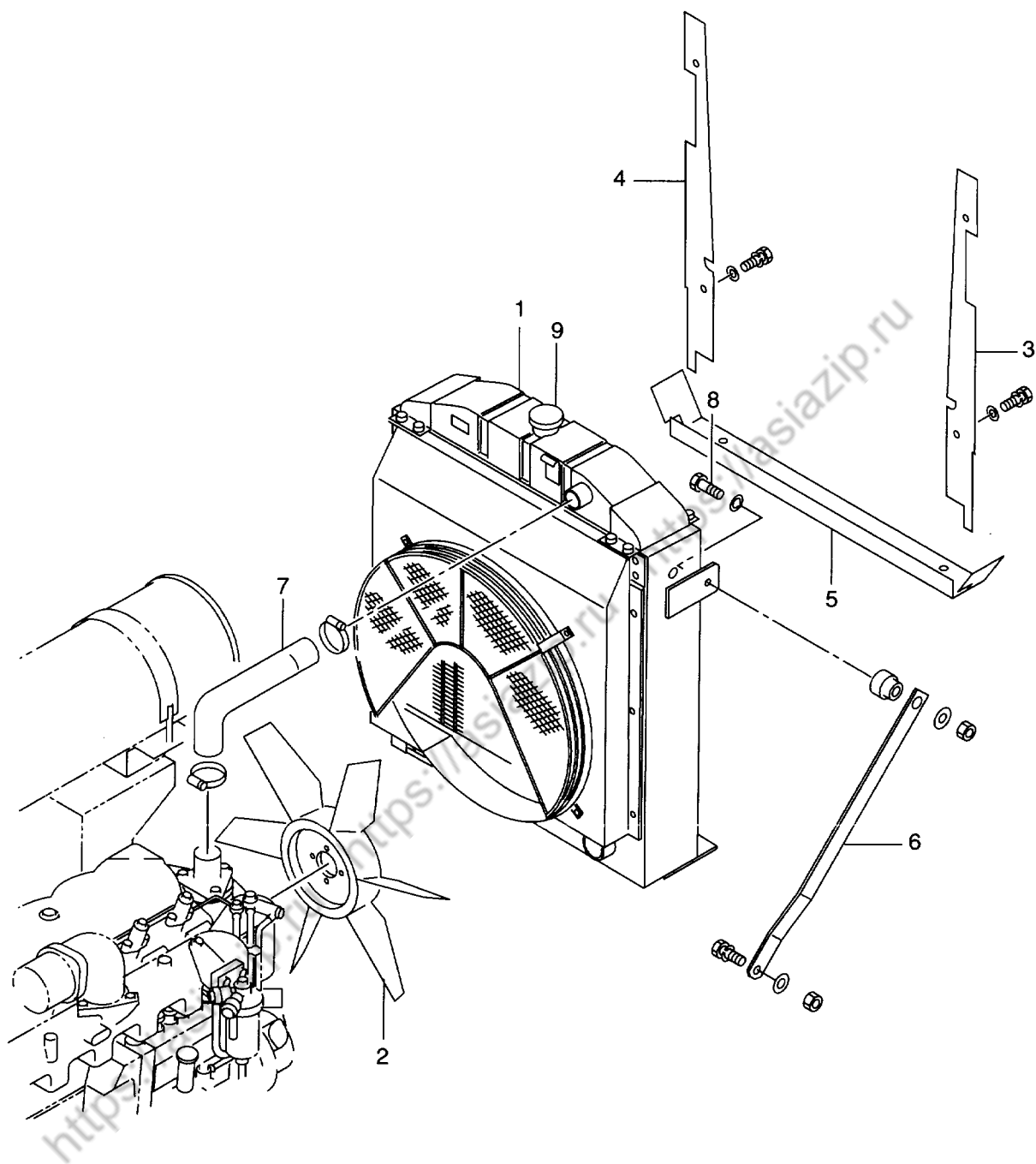
FIG. 5 DUST PROOF RADIATOR (DPR-648) (-2100) (OP) 防塵ラジエータ
