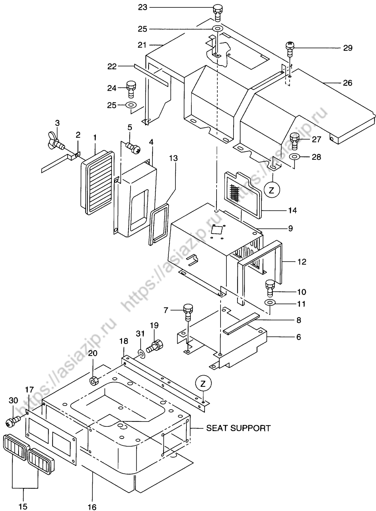
FIG. 151 AIR CONDITIONER (2/2) (-2100) エアコンディショナ
