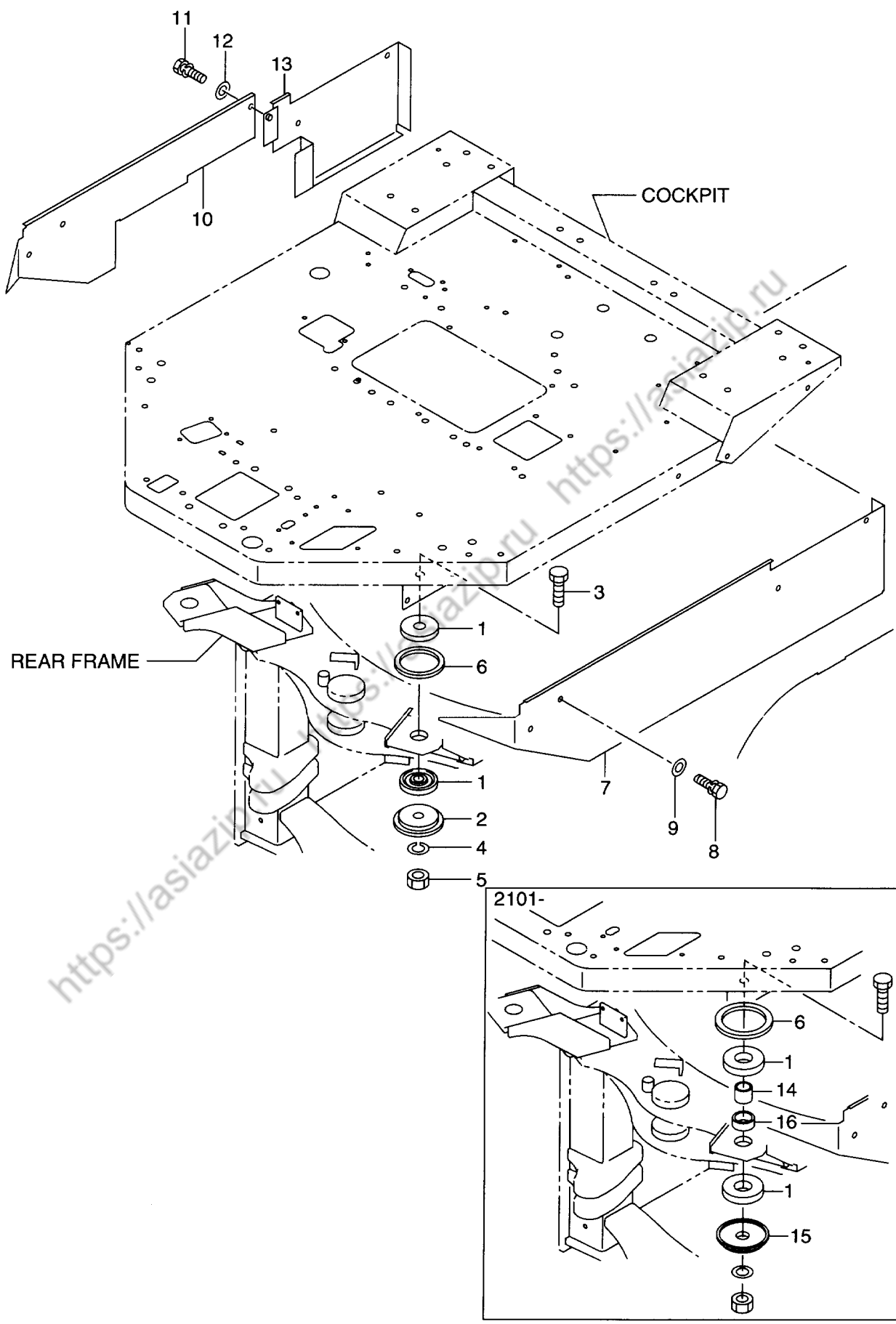
FIG. 74 COCKPIT MOUNT コックピットマウント
