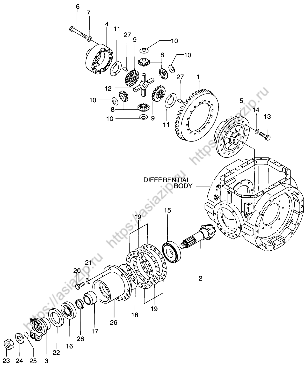
FIG. 51 DRIVE AXLE - REAR (3/3) ドライブ アクスル(リヤー)
