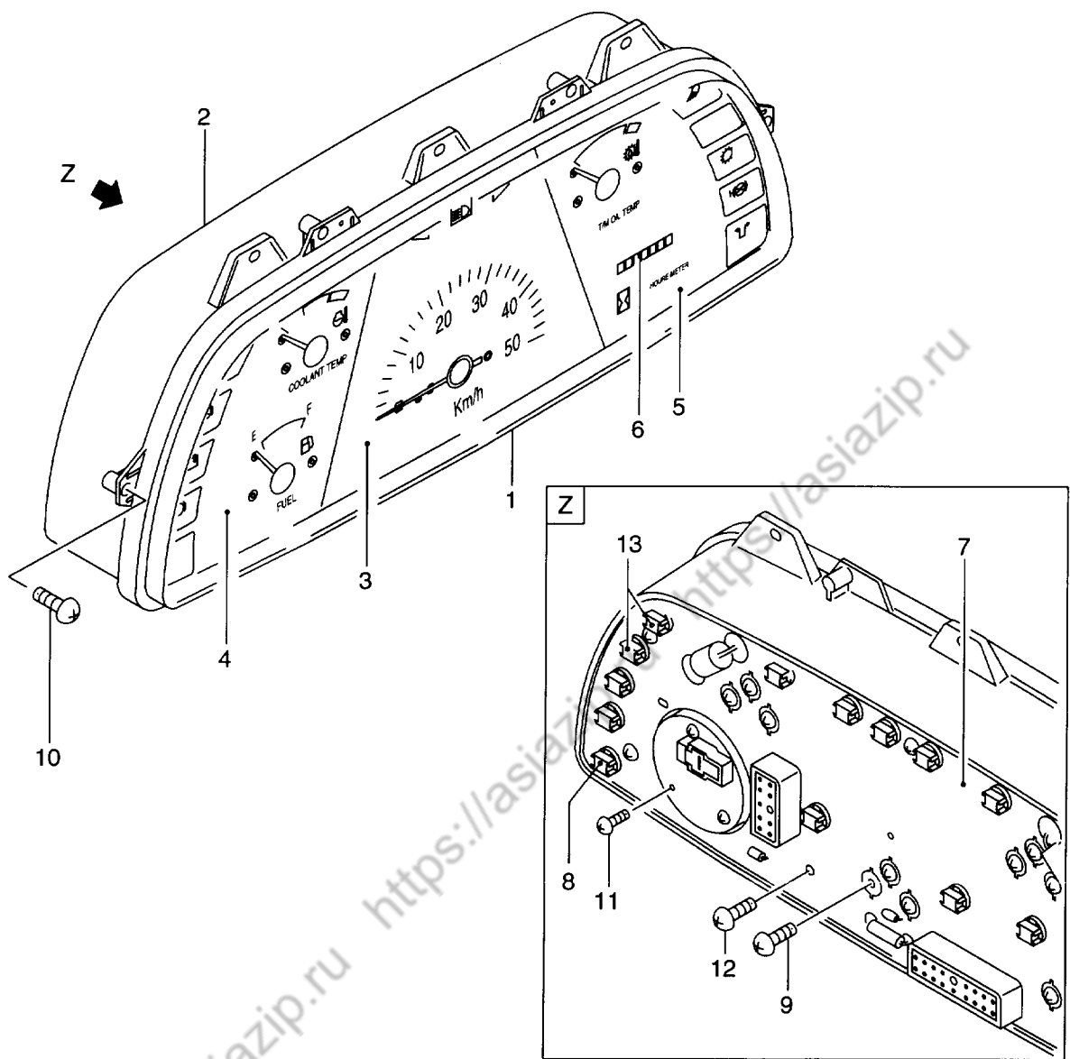
FIG. 16 CLUSTER METER クラスタメータ
