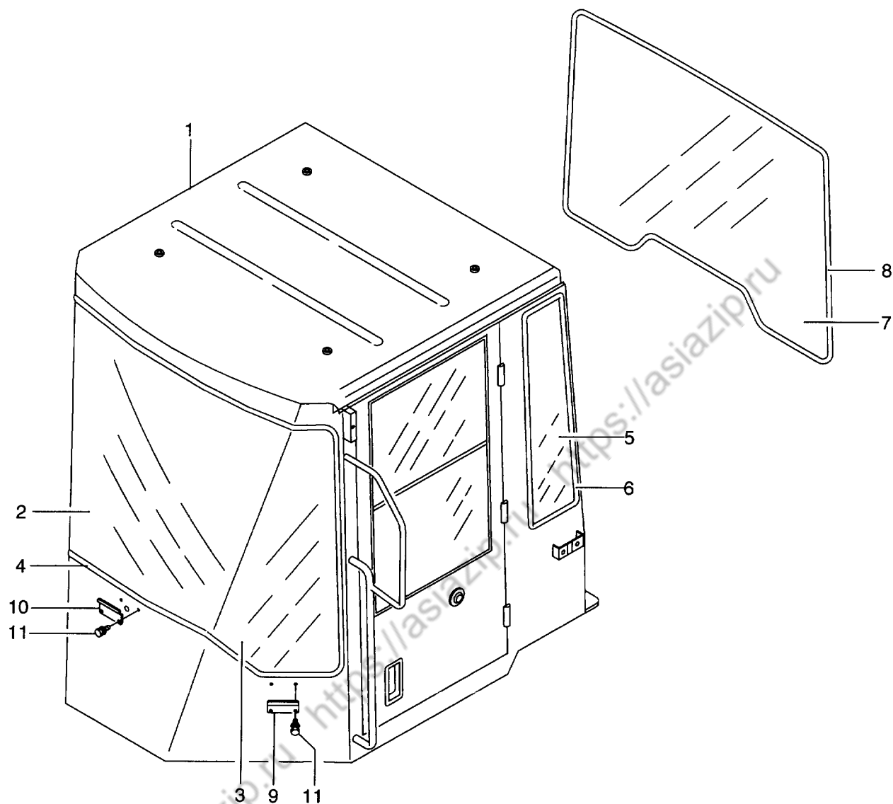
FIG. 95 LOW CAB (LCB150-648) (OP) ロ-キャブ
