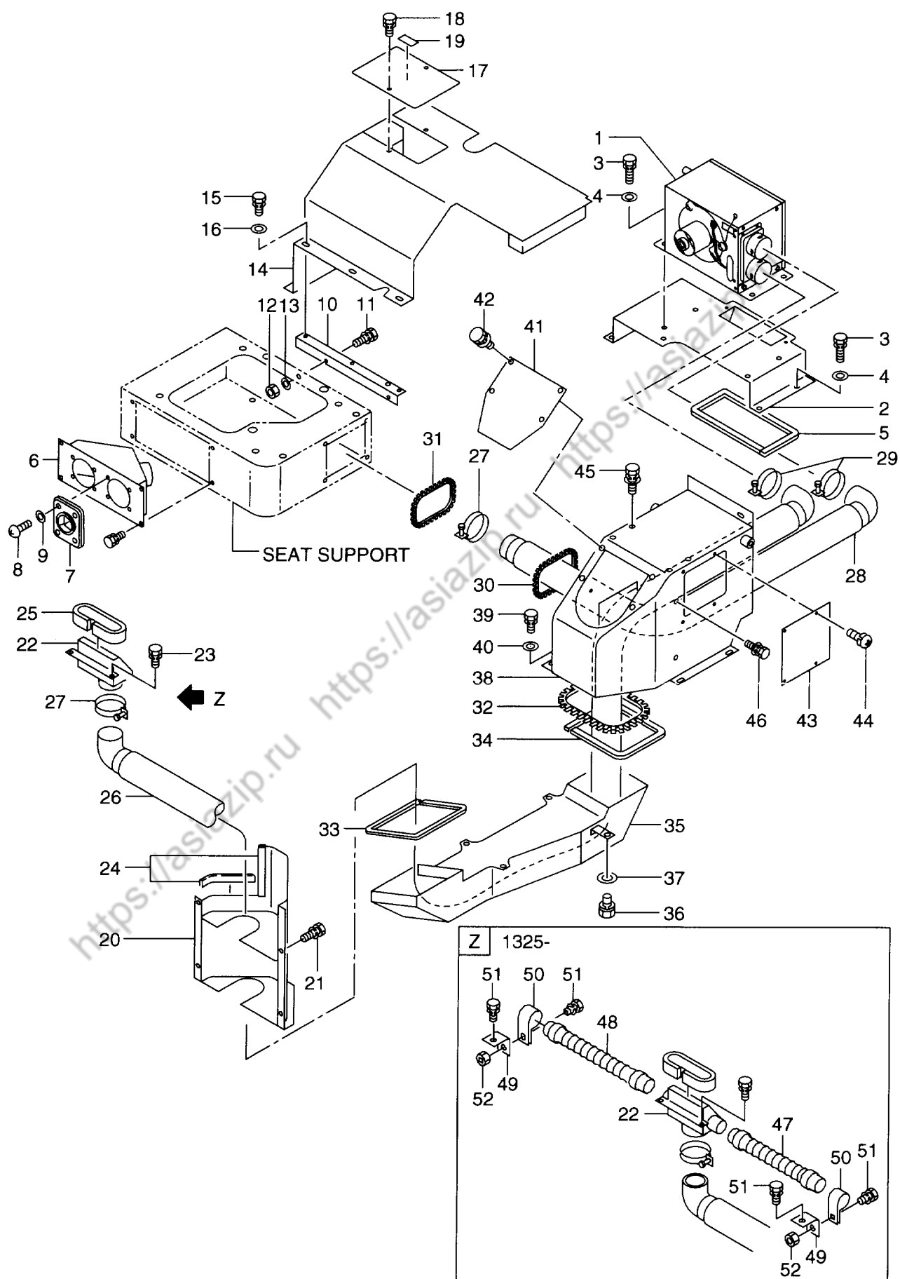
FIG. 28 HEATER (HR400A-648) (OP) ヒータ
