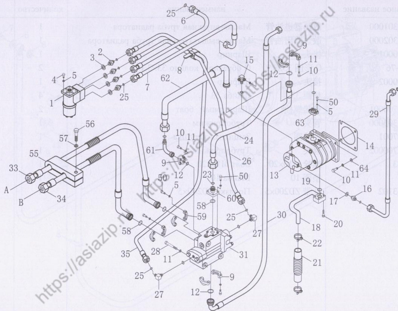
图 46-1 转向液压系统(一) Поворотная гидронасосная система ( I )
