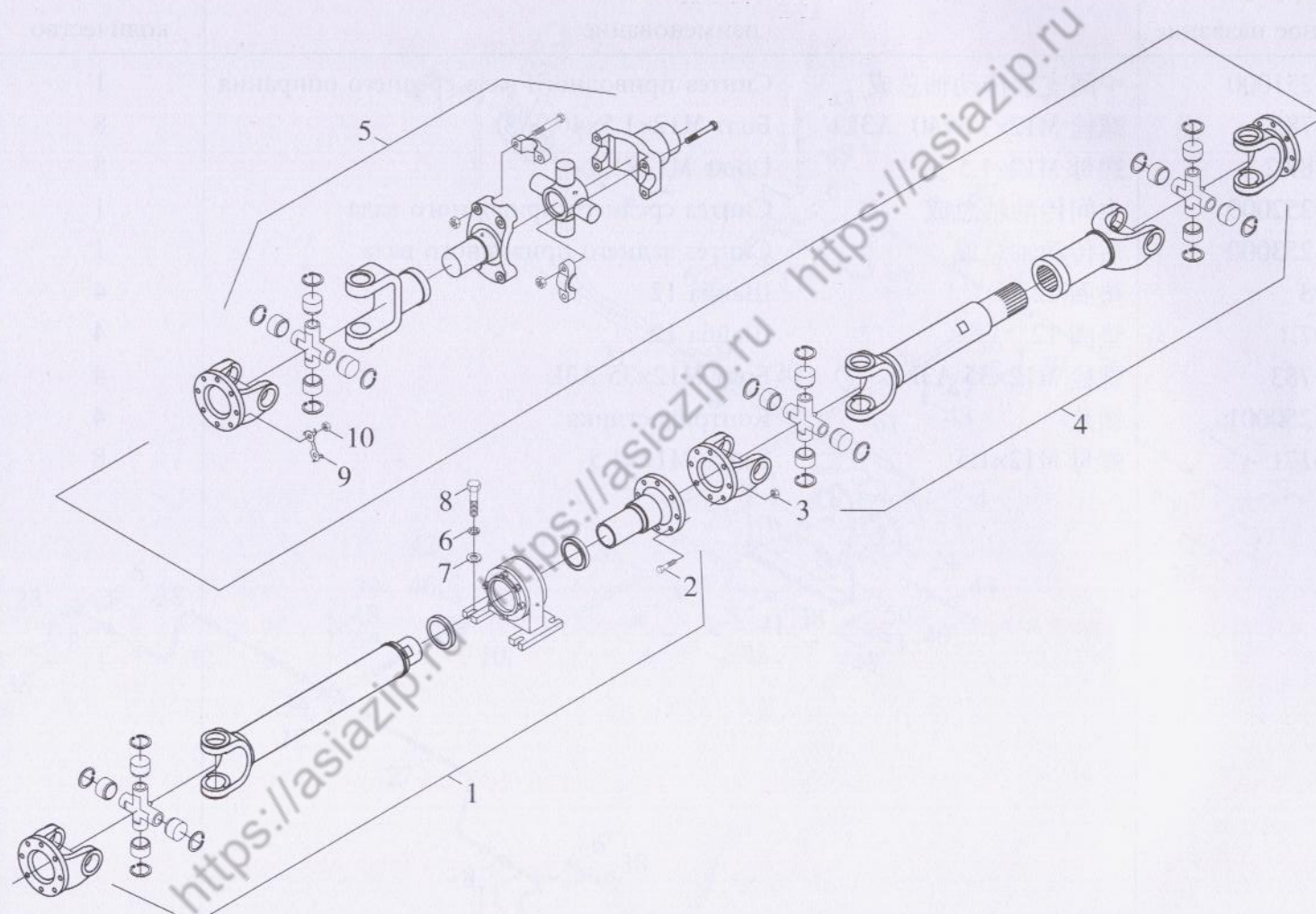
图 42 传动轴总成 Сбор передаточного вала
