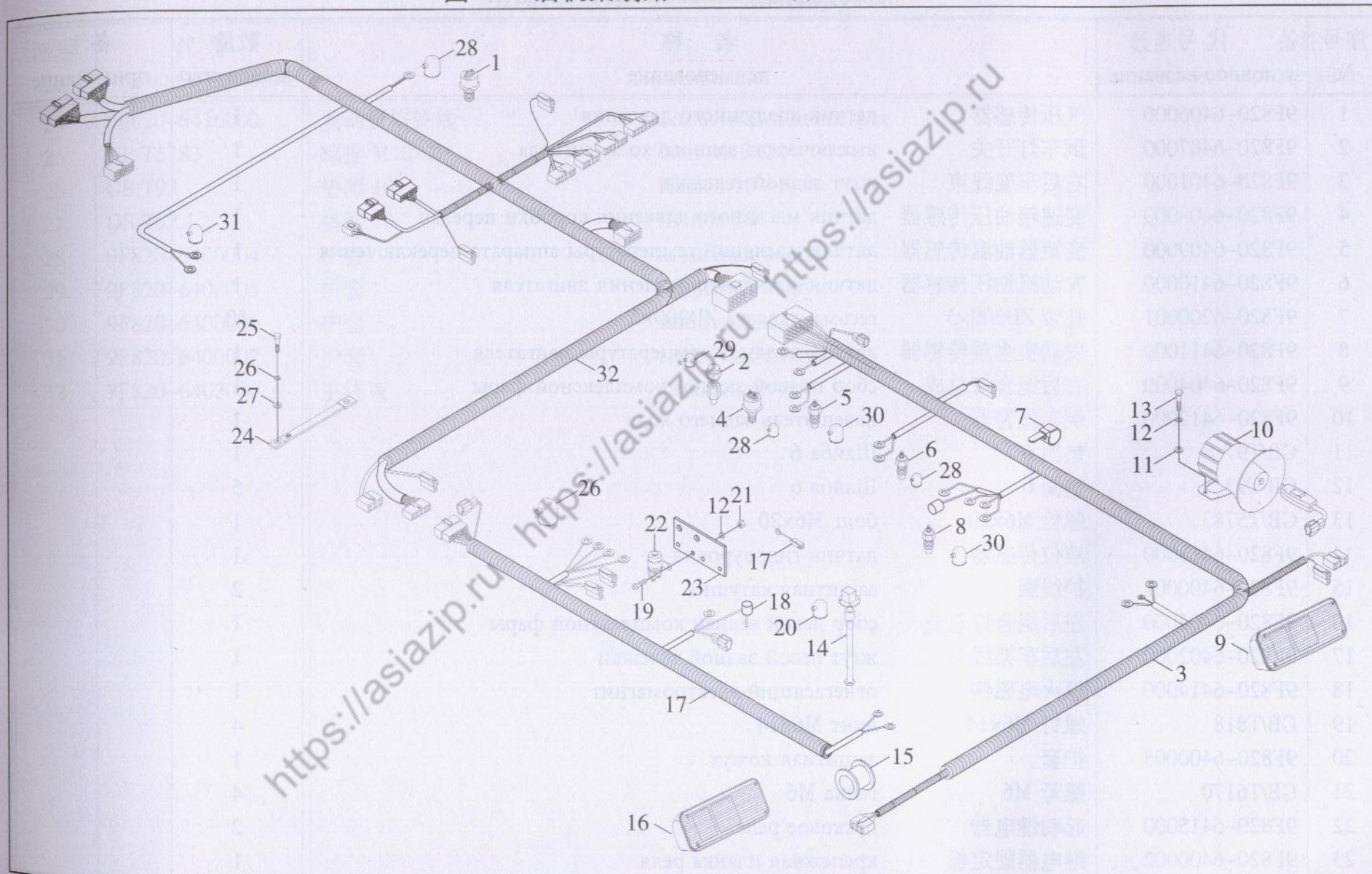
图 25 后机架线路 Линия заднего кyeti
