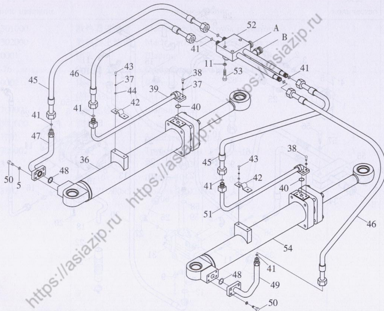
图 64-2 转向液压系统(二) Поворотная гидронасосная система ( II )
