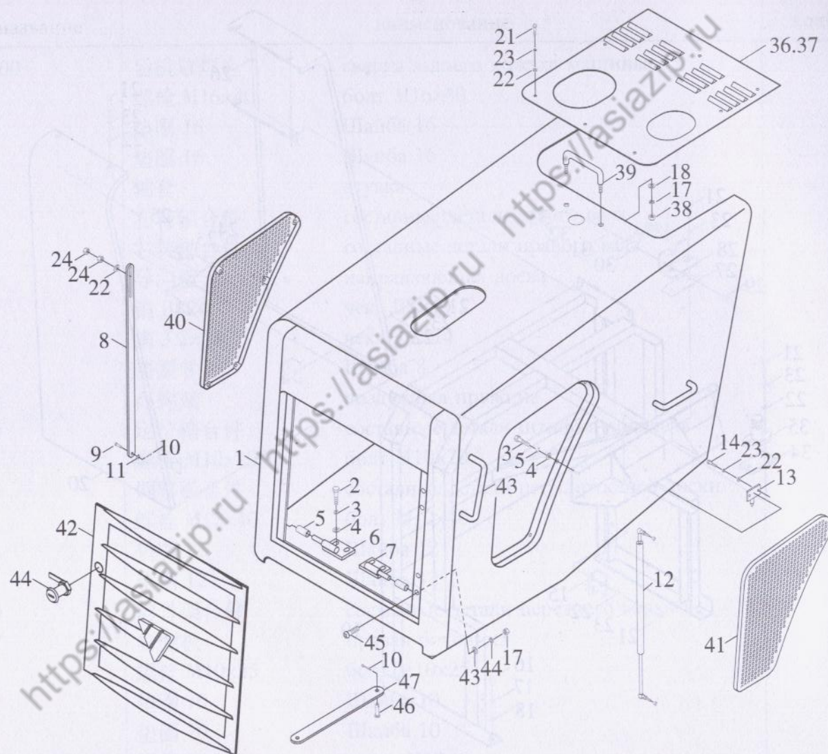
图 17-1 护罩总成(一) Сбор защитного кожуха ( I )
