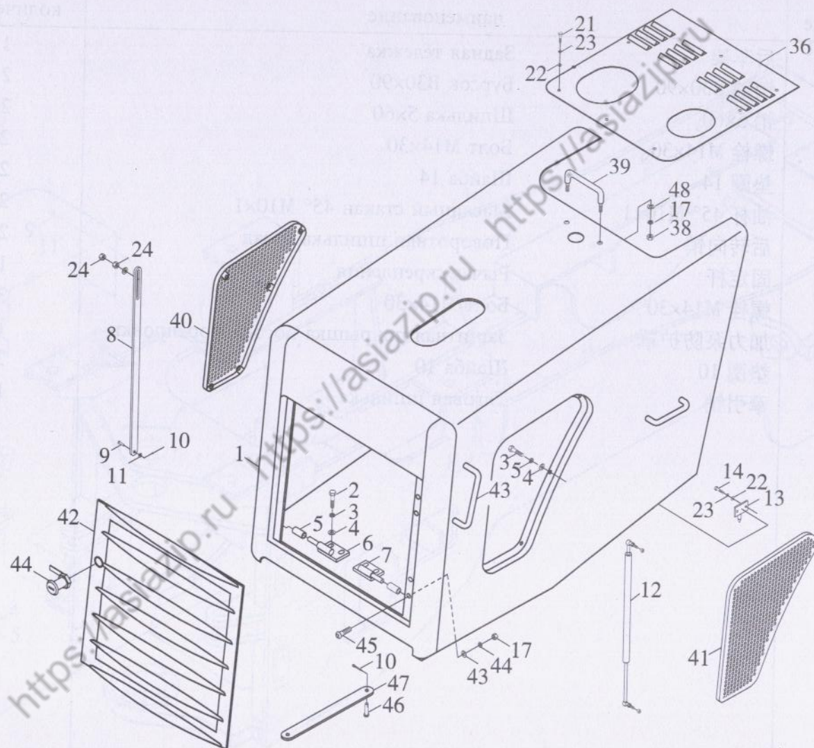
图 35-1 护罩总成(一) Сбор защитной рубашки (I)
