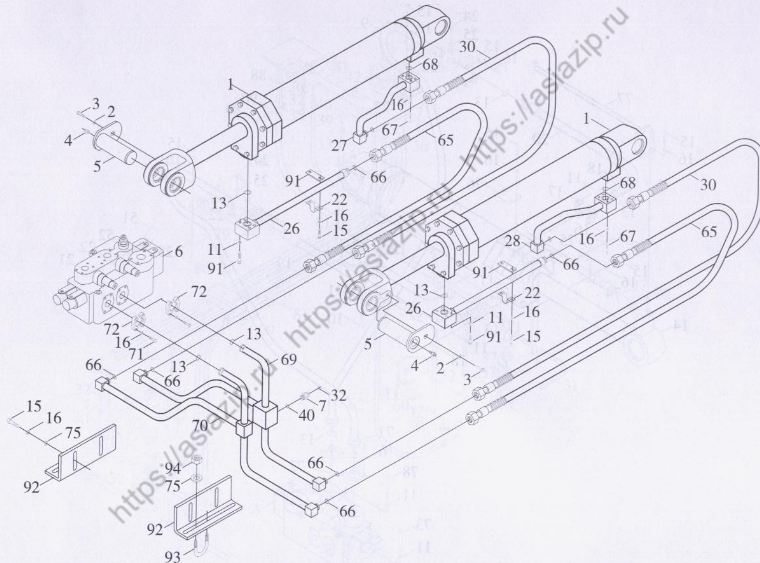
图 75-1 工作装置液压系统(一) Гидравлическая система рабочей аппаратуры ( I )
