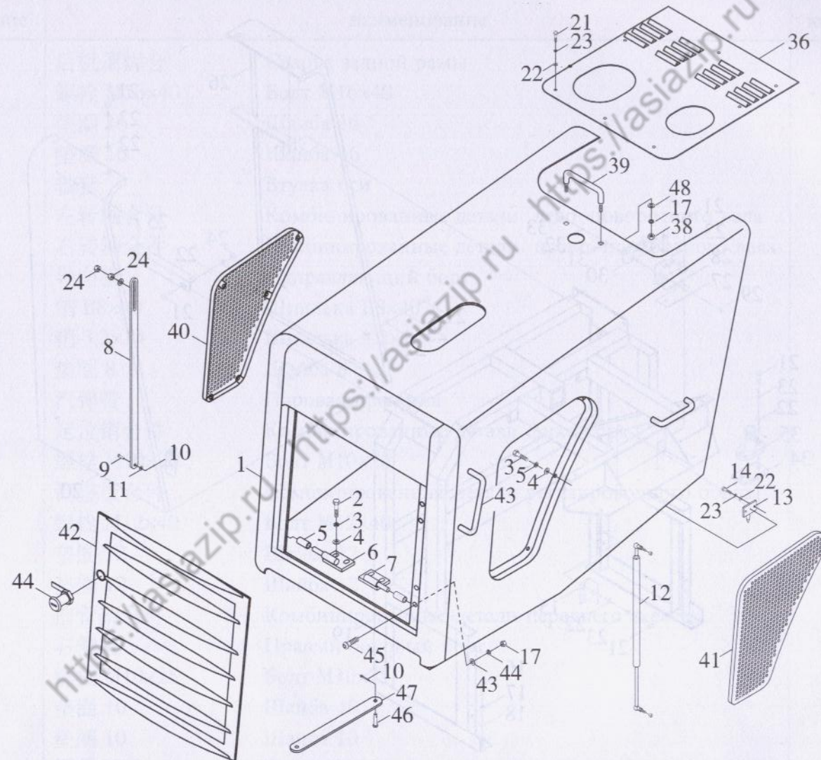
图 62-1 护罩总成(一) Сбор защитного кожуха ( I )
