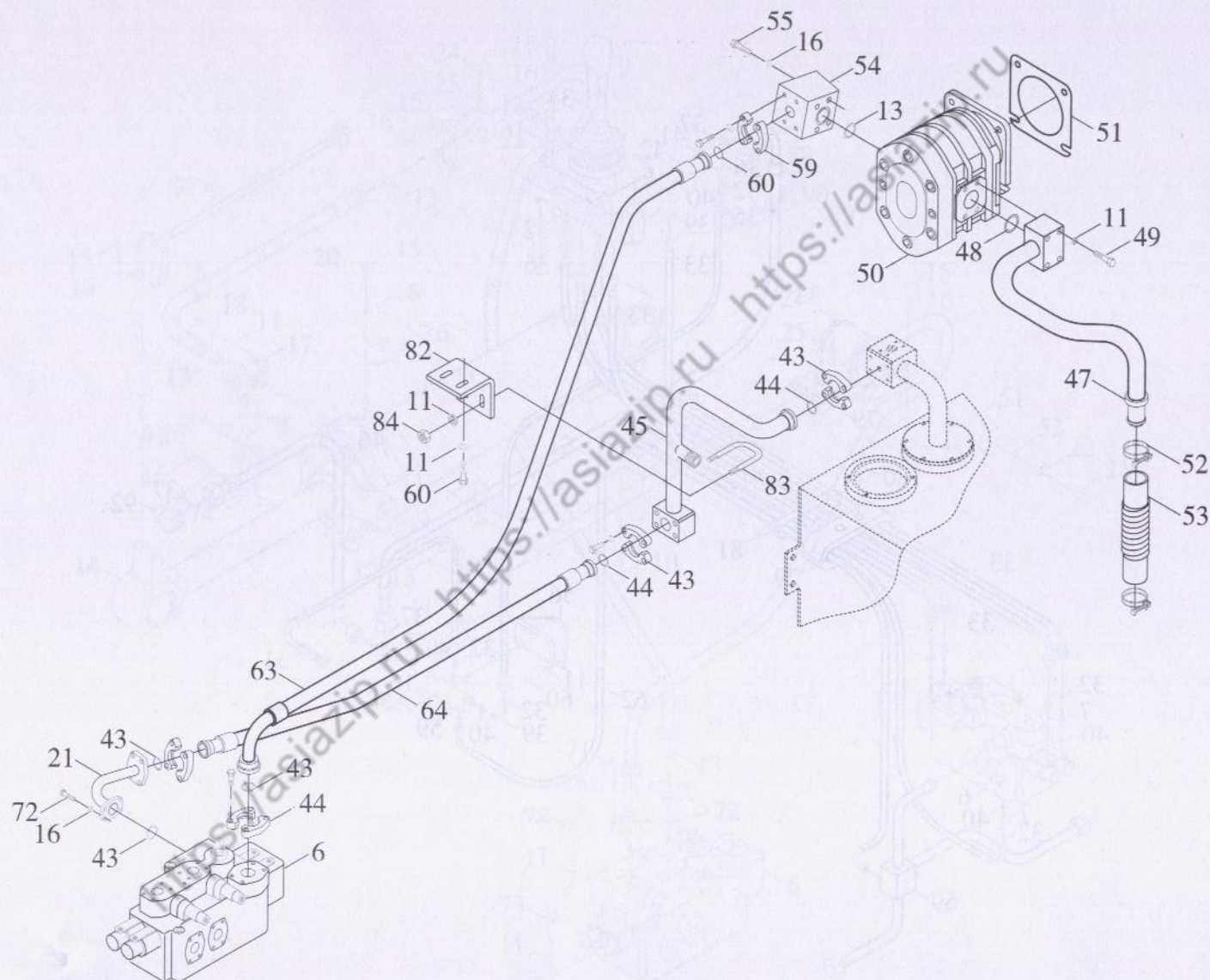
图 75-4 工作装置液压系统(四) Гидравлическая система рабочей аппаратуры (IV)
