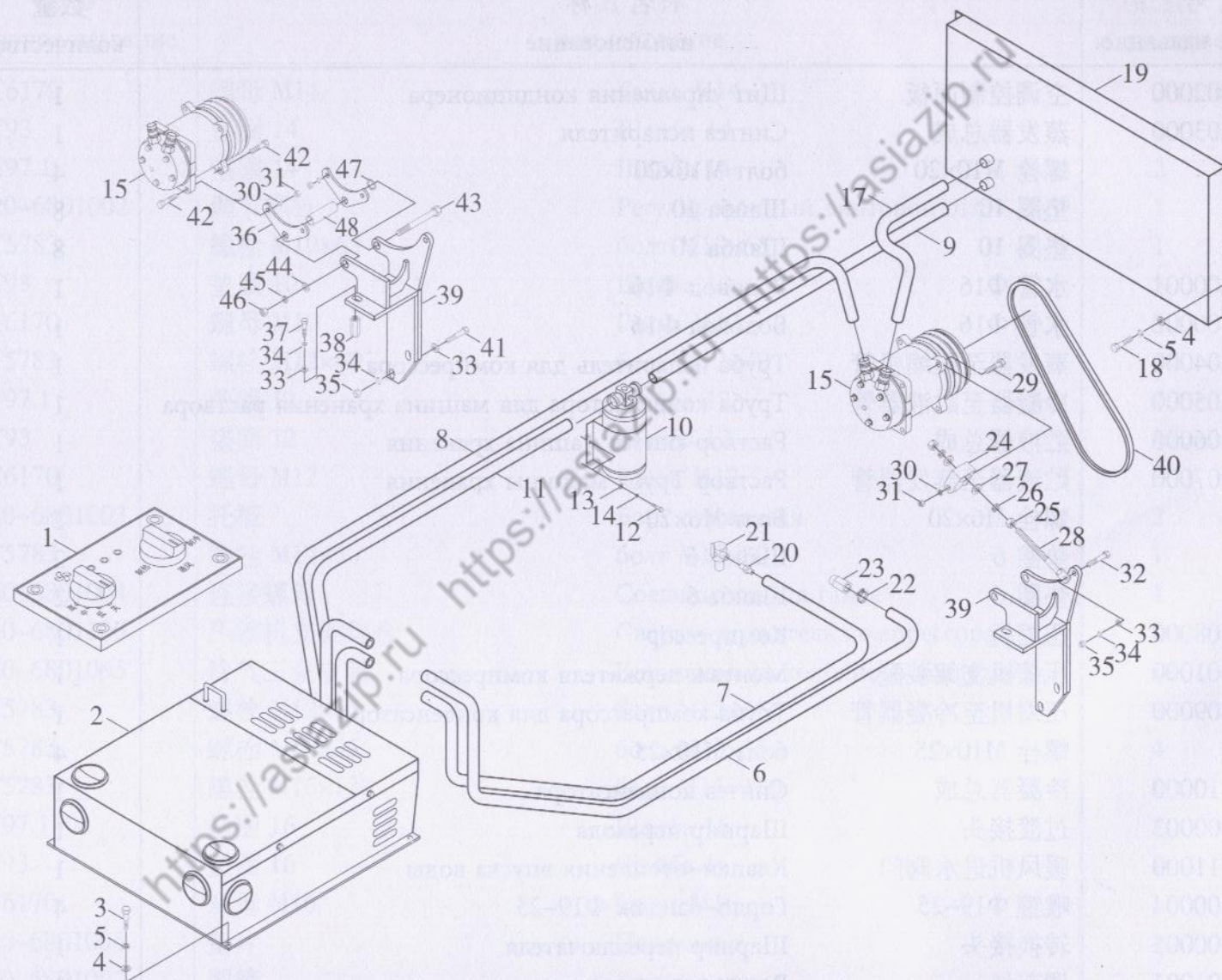
图 28 空调系统 Система кондиционера
