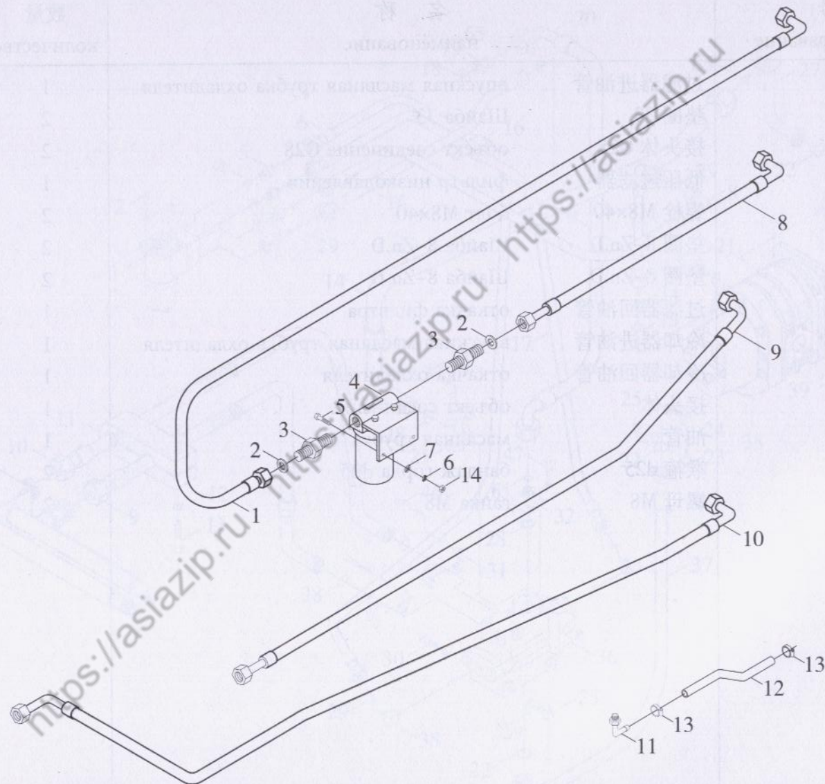
图 18 传动油路系统 Система передаточного масляного провода
