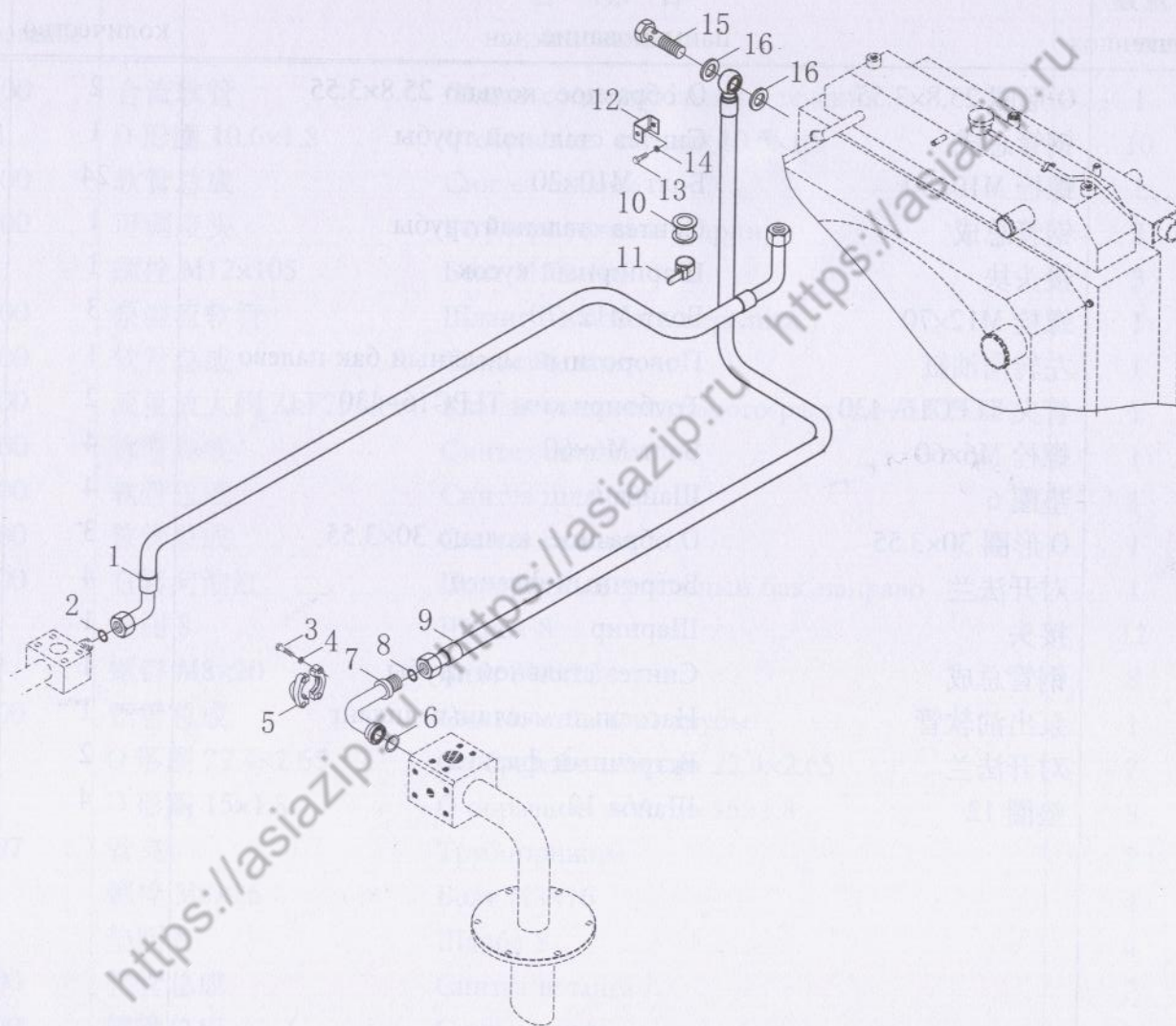
图 65 液压油散热系统 Гидронасосная масляная тепло-отводящая система
