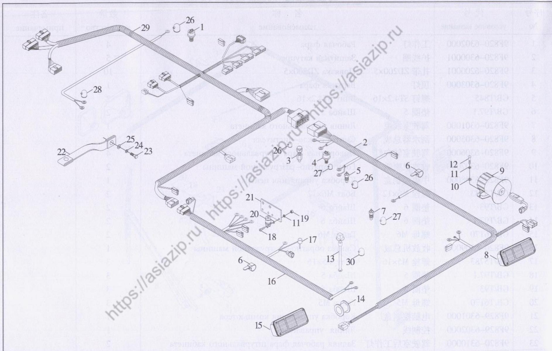
图 68 后机架线路 Линия заднего кyeti
