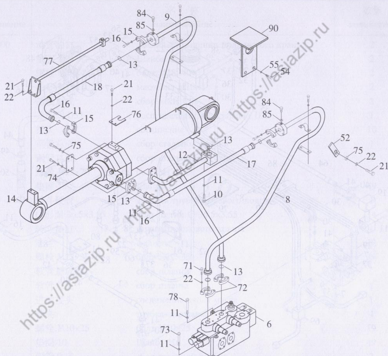
图 22-2 工作装置液压系统(二) Гидронасосная система работающей аппаратуры ( II )
