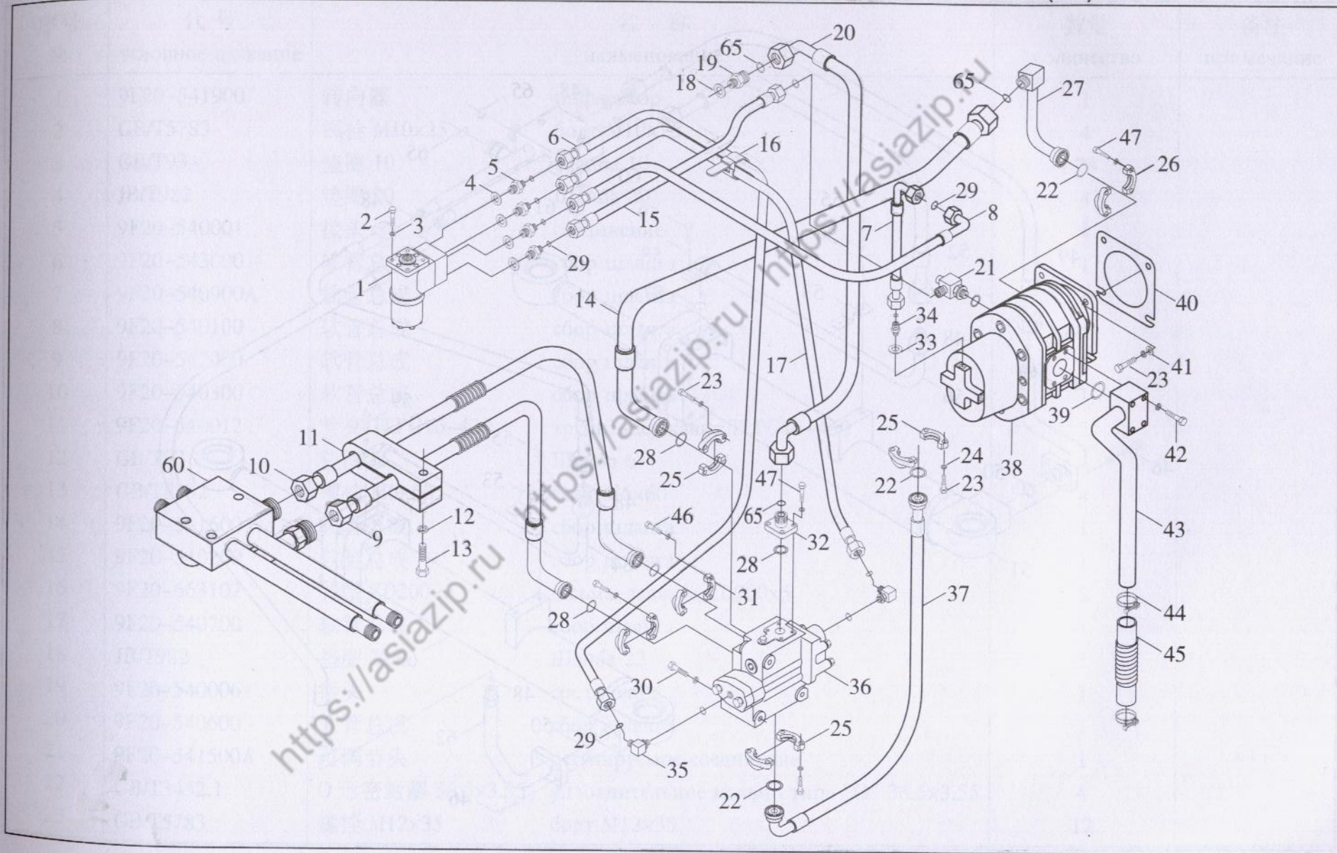
图 19-1 转向液压系统(一) Поворотная гидронасосная система ( I )
