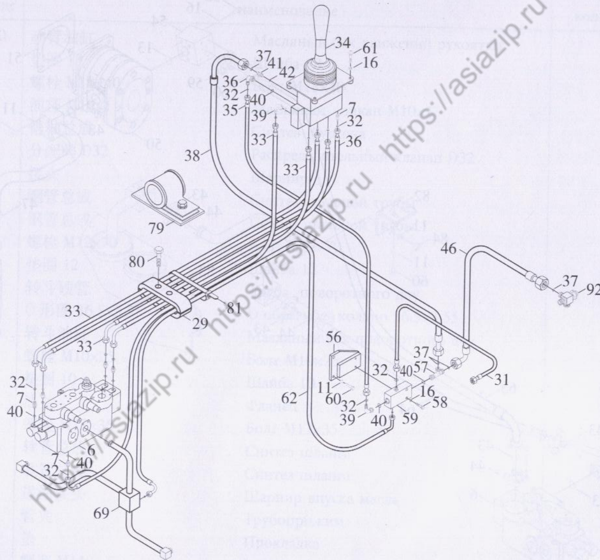
图 72-3 工作装置液压系统(三) Гидравлическая система рабочей аппаратуры ( III )
