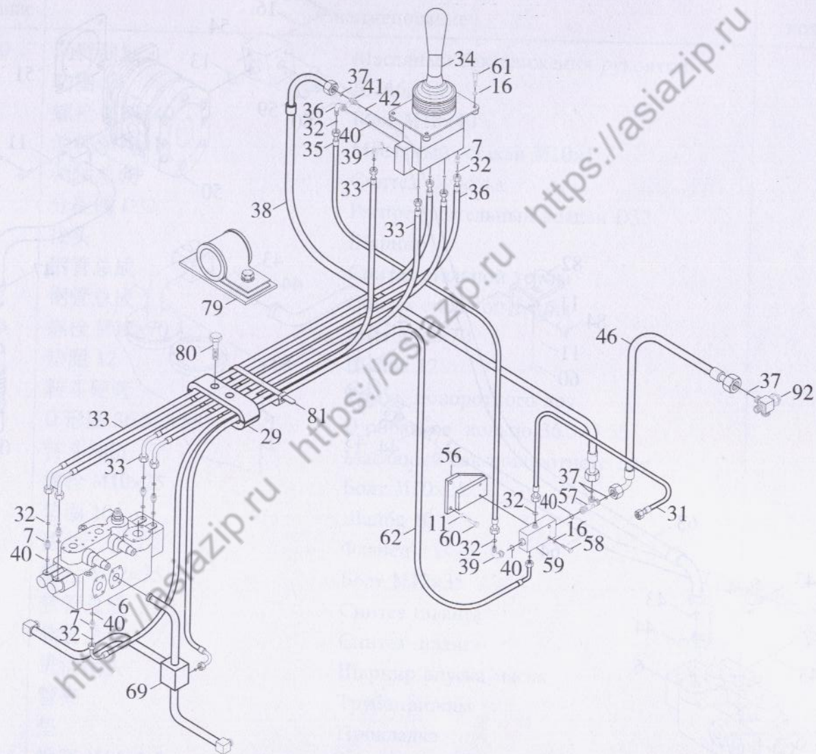
图 75-3 工作装置液压系统(三) Гидравлическая система рабочей аппаратуры ( III )
