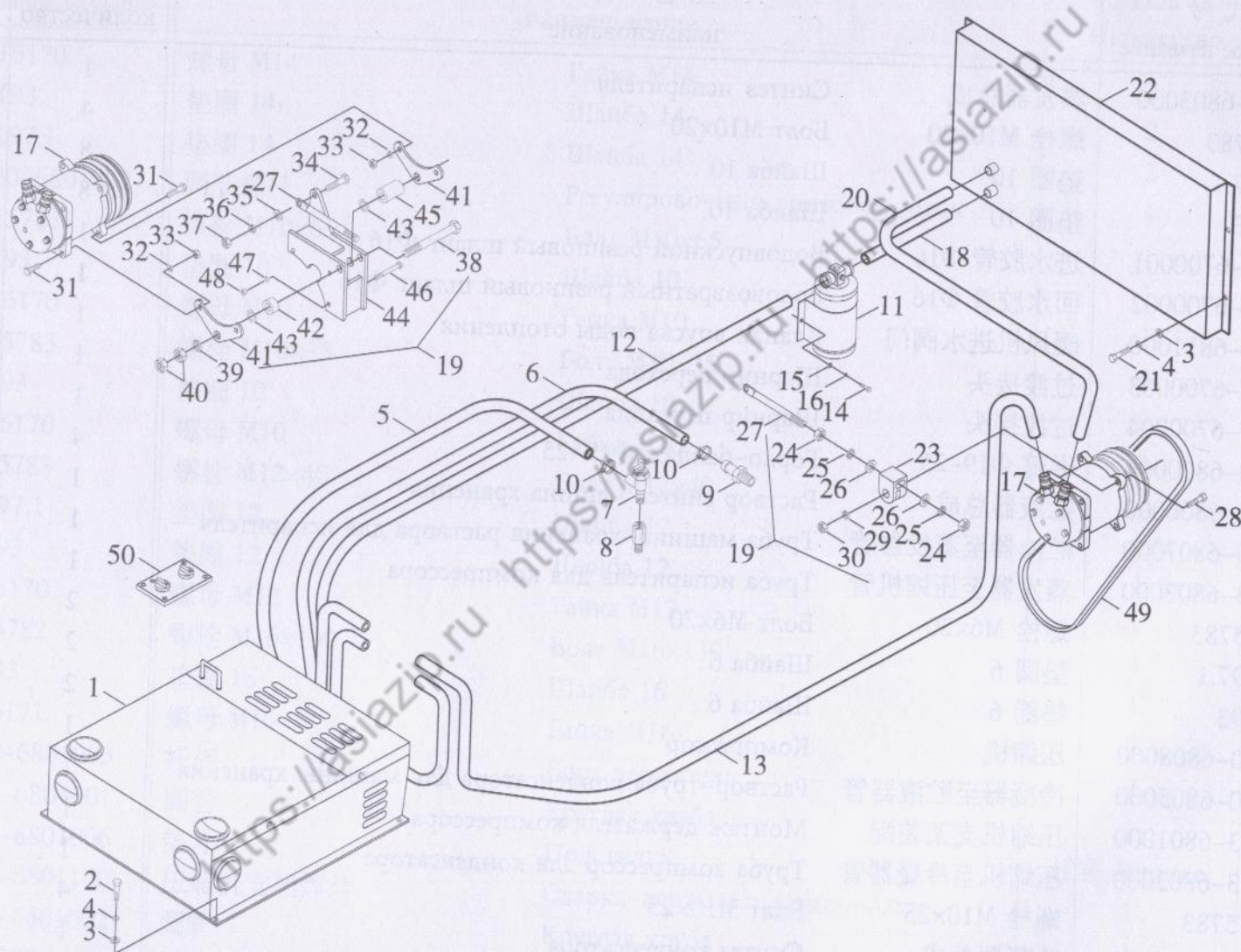
图 70 空调系统 Система кондиционера
