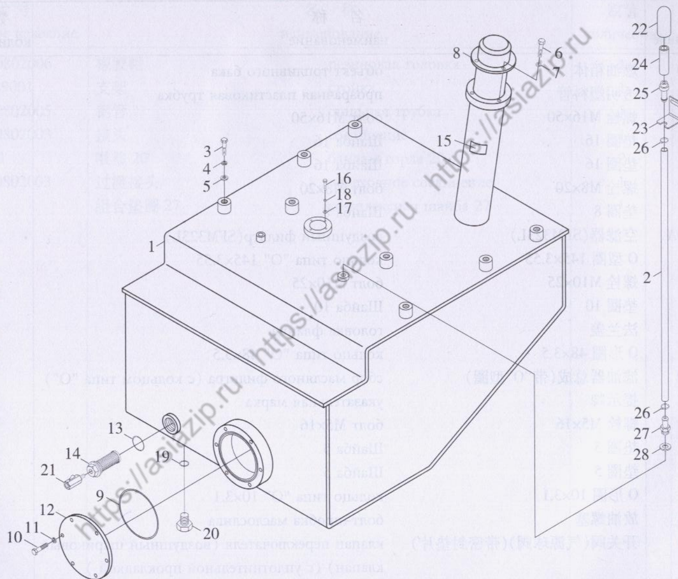
图 4 燃油箱 Топливный бак
