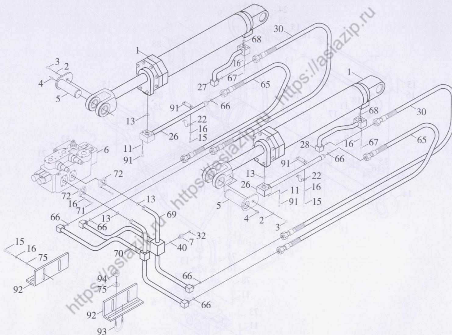
图 72-1 工作装置液压系统(一) Гидравлическая система рабочей аппаратуры ( I )
