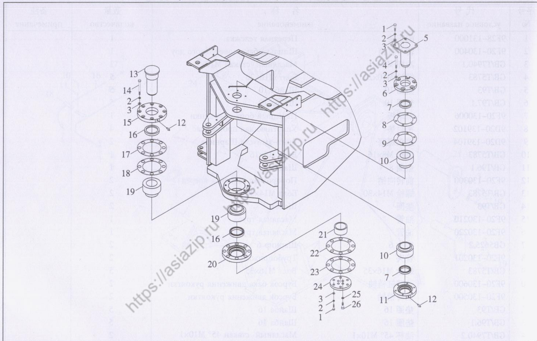
图 55-2 车架(铰接总成) Тележка (синтез шарнирного соединения)
