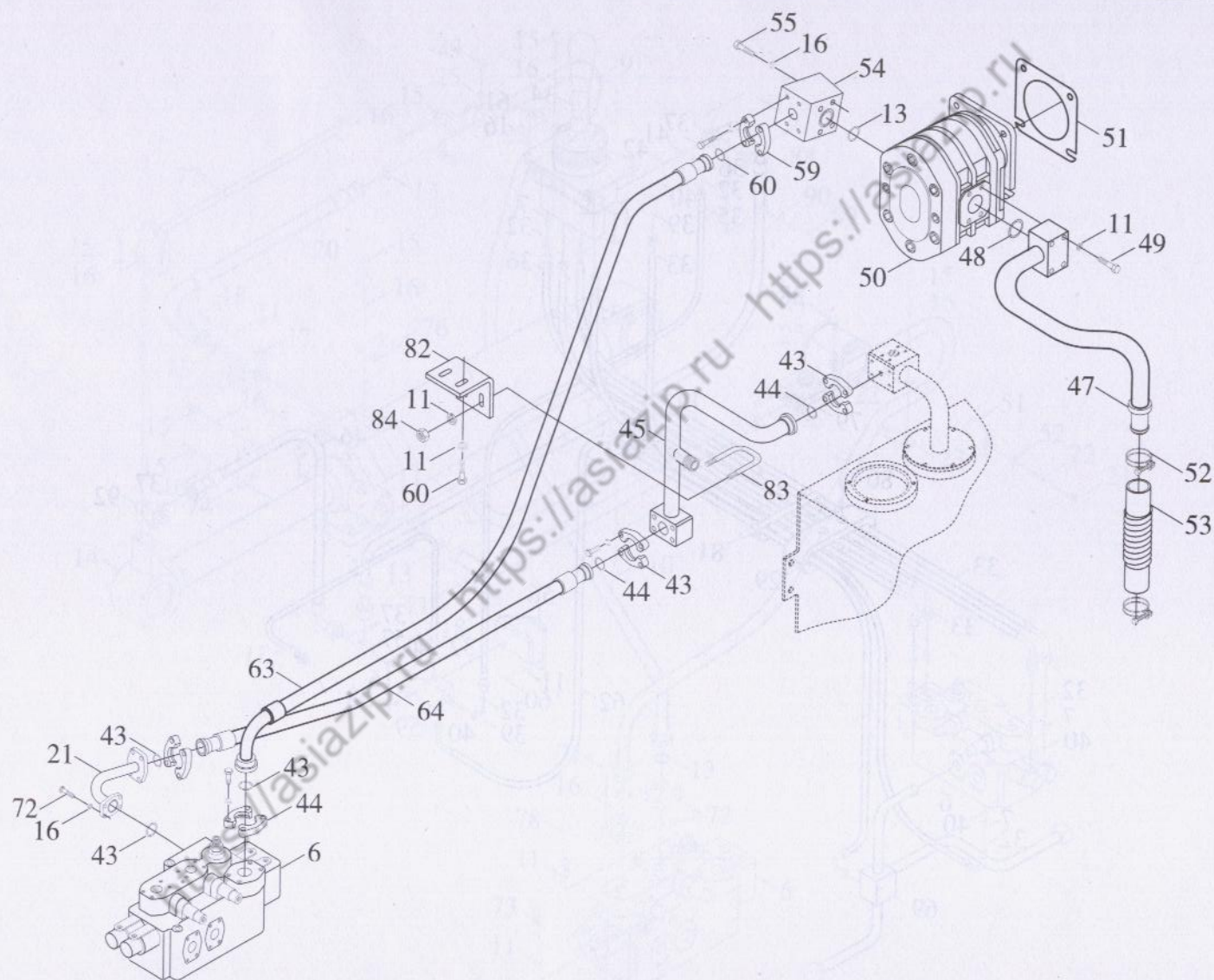
图 78-4 工作装置液压系统(四) Гидравлическая система рабочей аппаратуры (IV)
