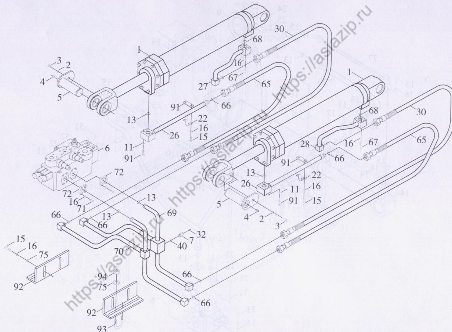
图 78-1 工作装置液压系统(一) Гидравлическая система рабочей аппаратуры ( I )
