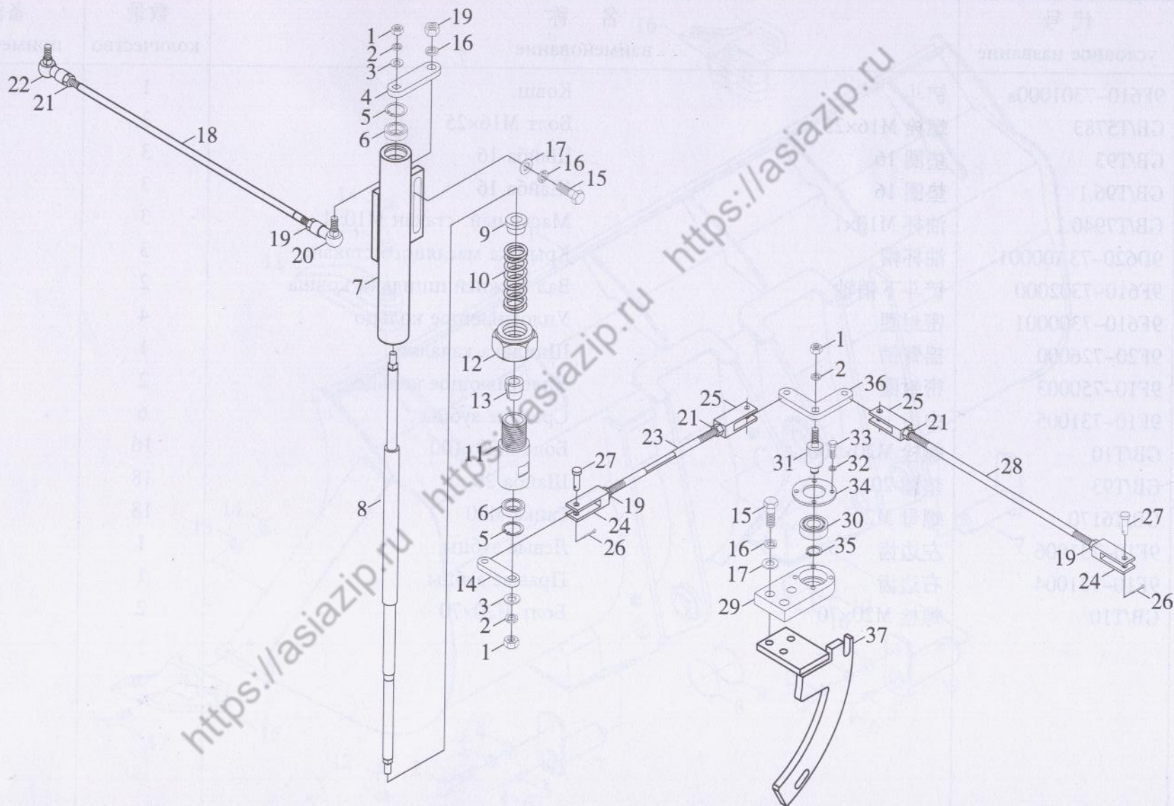
图 31 变速操纵系统 Система управления скоростями
