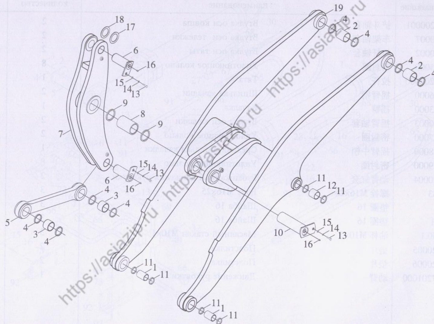
图 71 连杆机构 Механизм соединительного рычага
