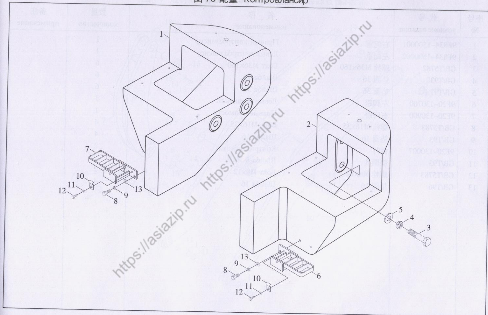
图 73 配重 Контрбалансир
