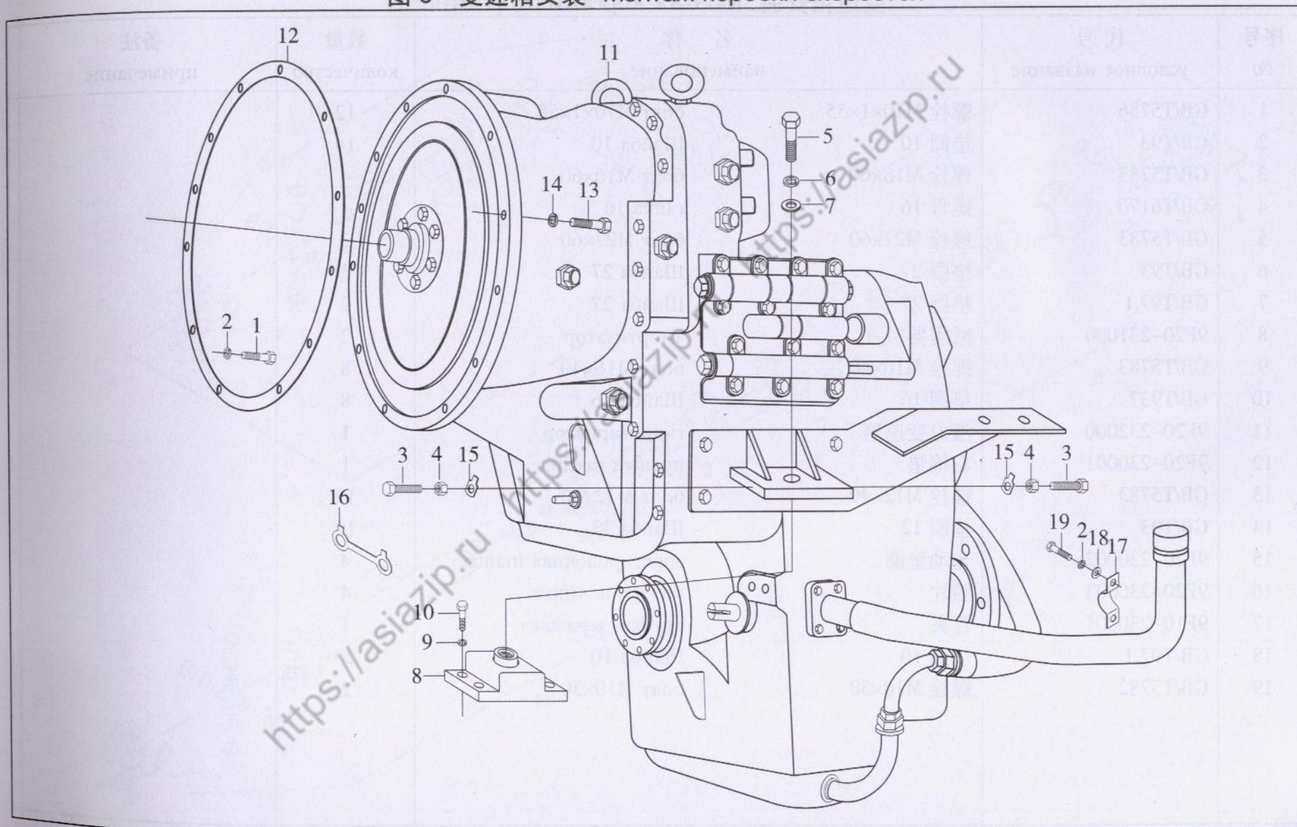
图6 变速箱安装 Монтаж коробки скоростей
