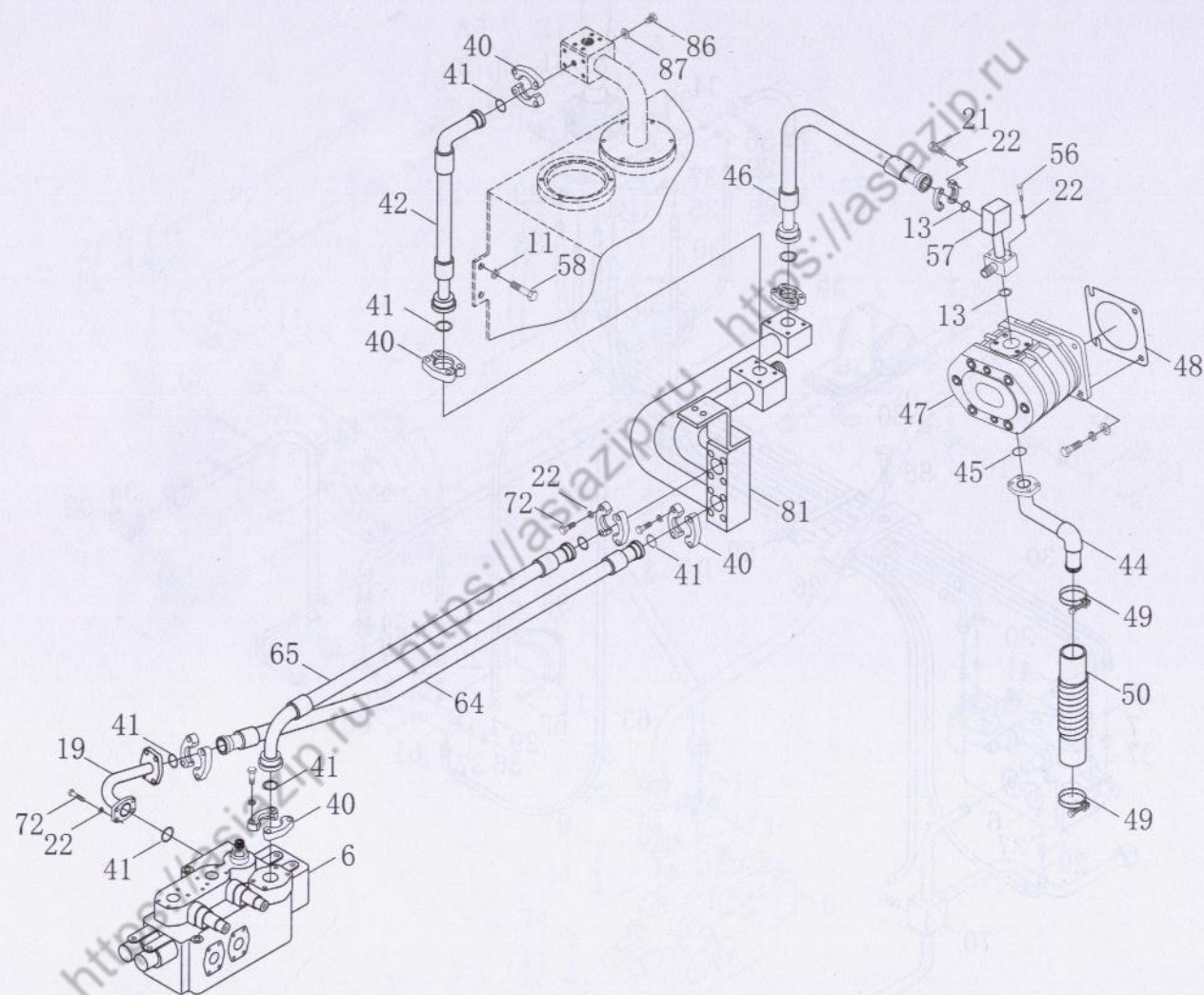
图 48-4 工作装置液压系统(四) Гидравлическая система рабочего аппарата (IV)
