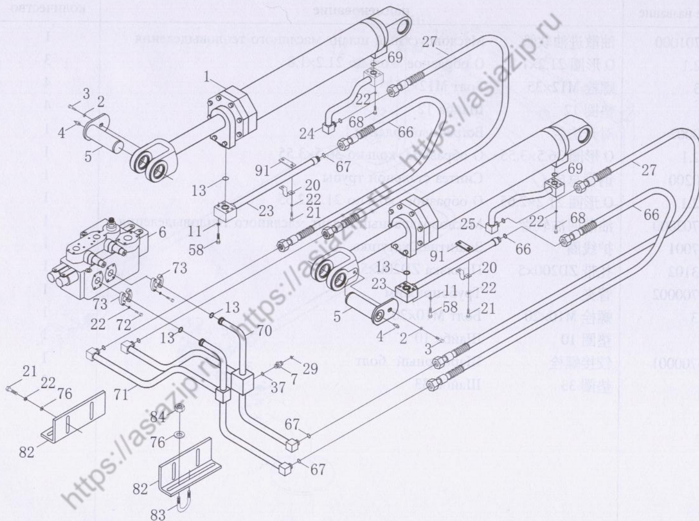
图 66-1 工作装置液压系统(一) Гидравлическая система рабочего аппарата ( I )
